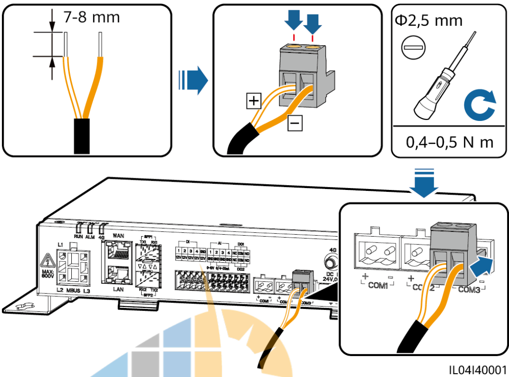
Abbildung 4-2 Anschließen eines RS485-Kommunikationskabels
