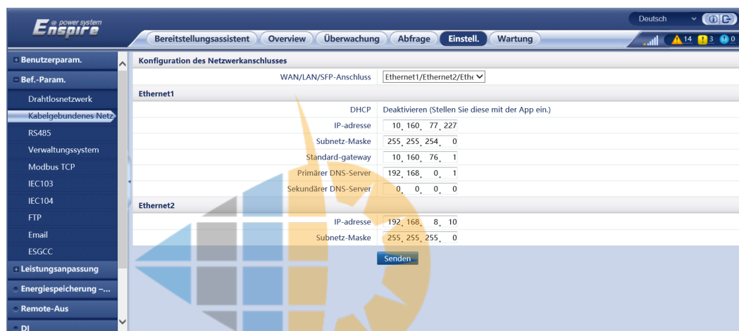
Abbildung 6-28 Einstellen der Parameter des kabelgebundenen Netzwerks
