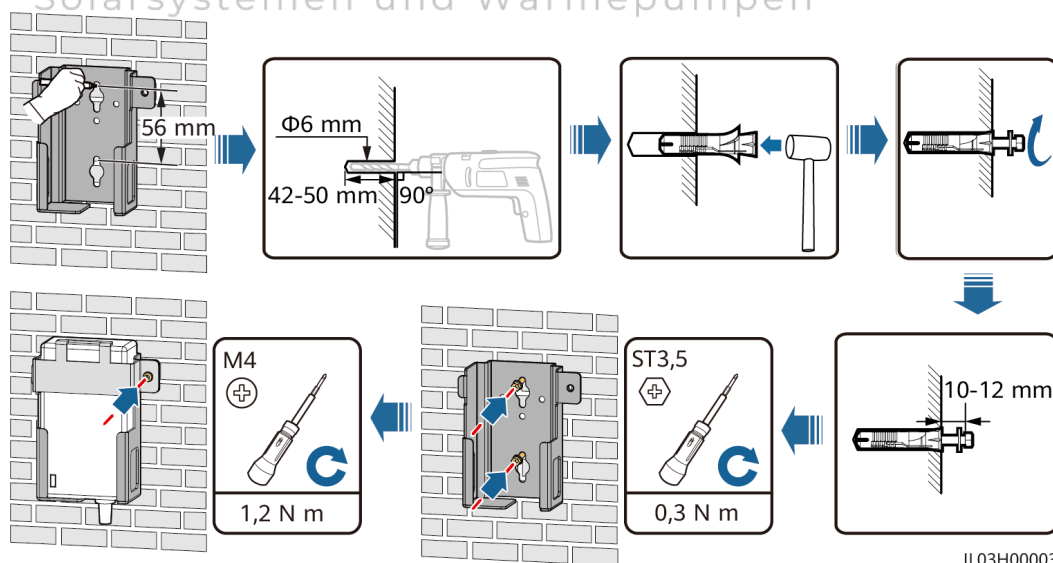
Abbildung 3-9 Wandmontage (Modus 1)
