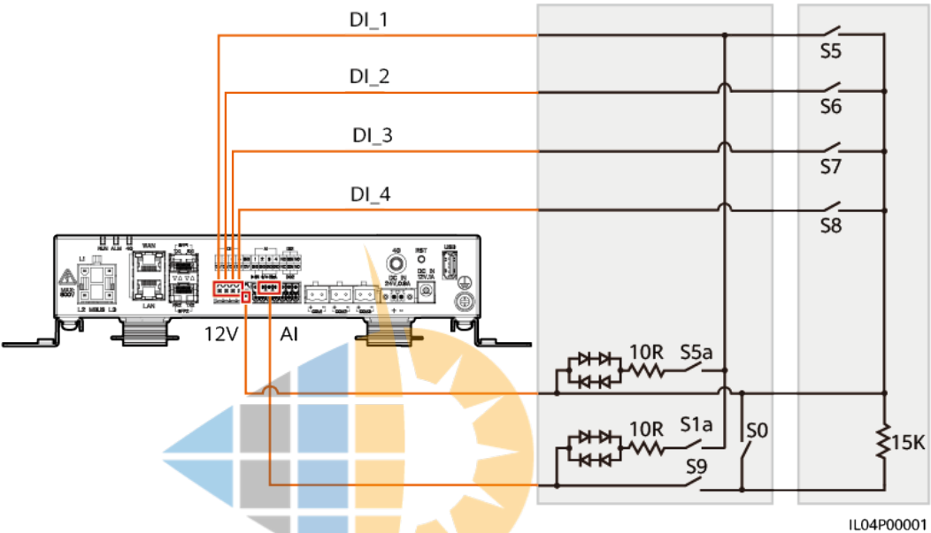
Abbildung 6-86 Schaltplan für die DRM-Funktion
