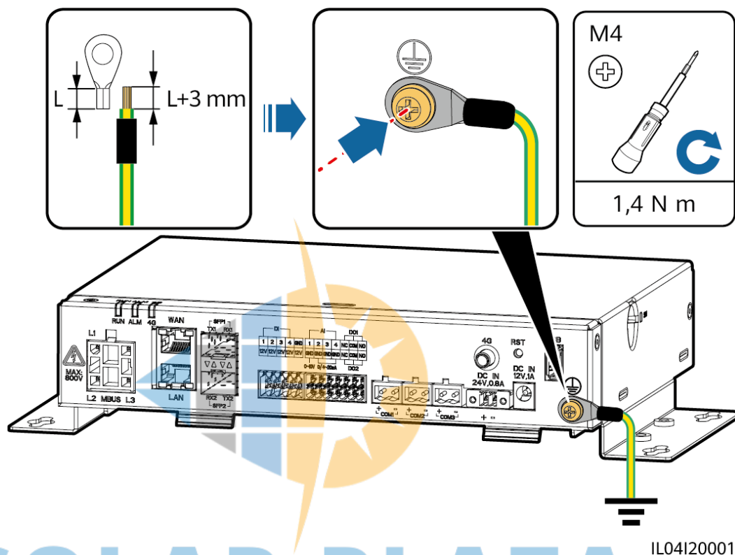
Abbildung 4-1 Anschließen eines PE-Kabels
