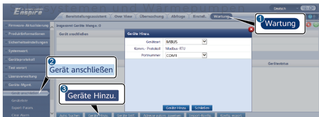
Abbildung 6-37 Einstellen der Zugriffsparameter für einen externen MBUS
