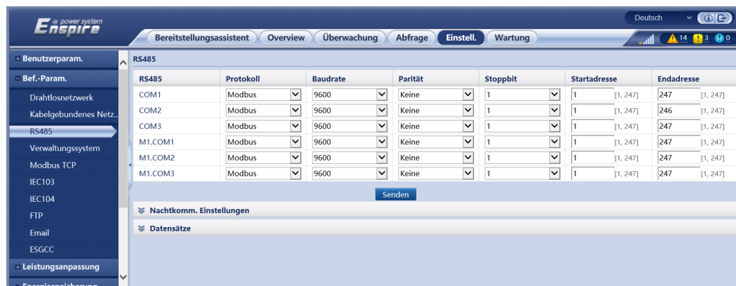
Abbildung 6-33 Einstellen von RS485-Parametern
