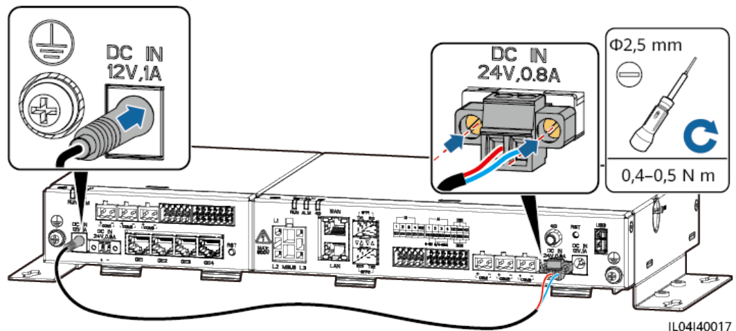
Abbildung 4-16 Anschließen des 12-V-Eingangsstromkabels
