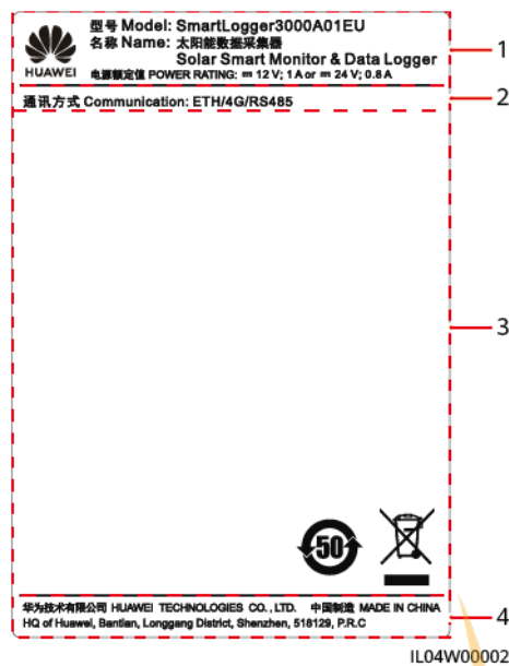
Abbildung 2-2 Typenschild
