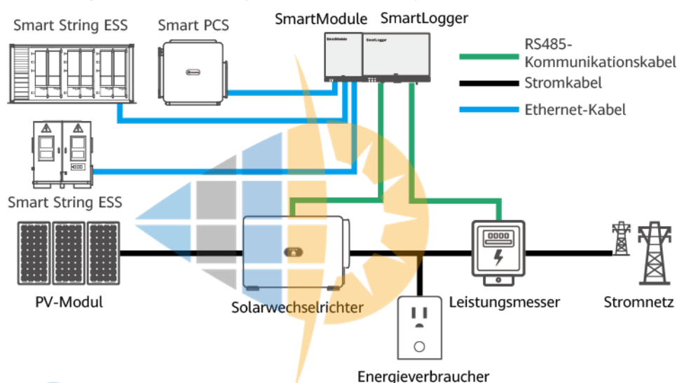
Abbildung 6-81 Netzwerkdiagramm (ohne Leistungsschalter)
