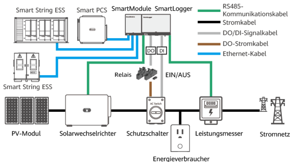
Abbildung 6-82 Netzwerkdiagramm (mit Leistungsschalter)
