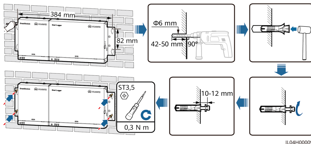
Abbildung 3-5 Wandmontage
