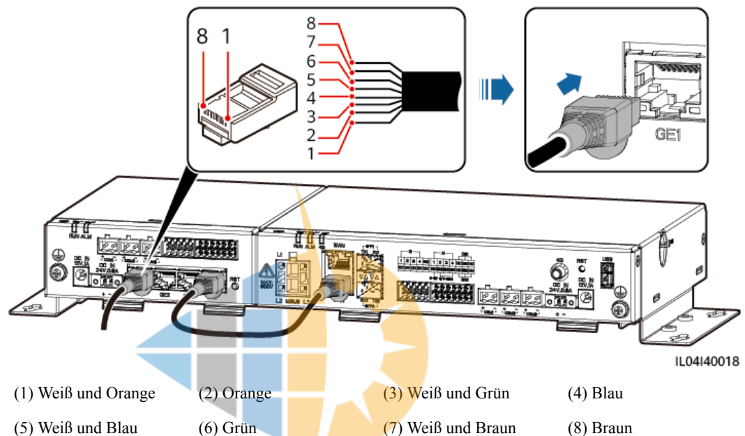
Abbildung 4-15 Anschließen des Ethernet-Kabels
