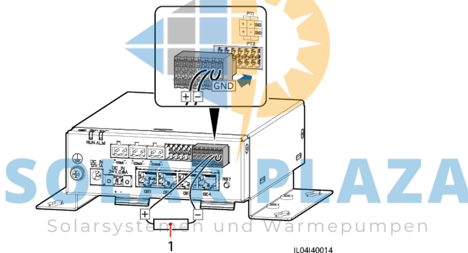
Abbildung 4-23 Anschließen an einen Zweileiter-PT100/PT1000
