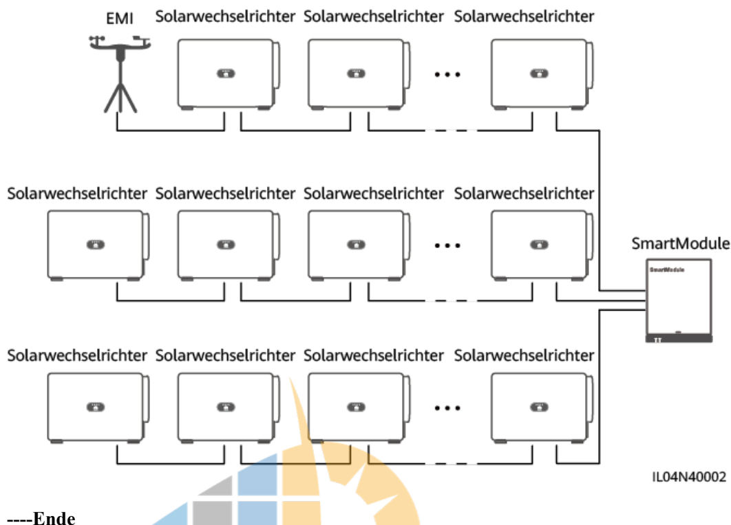
Abbildung 4-18 Kaskadierende Verbindung
