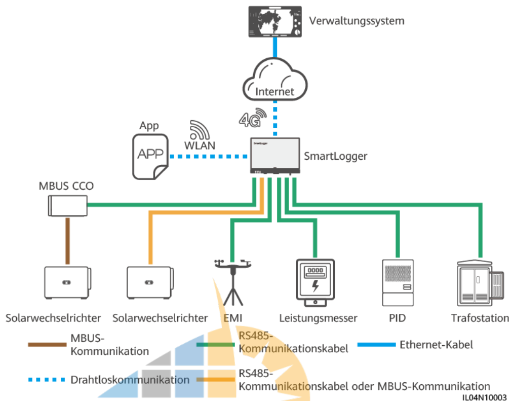
Abbildung 2-5 4G-Netz
