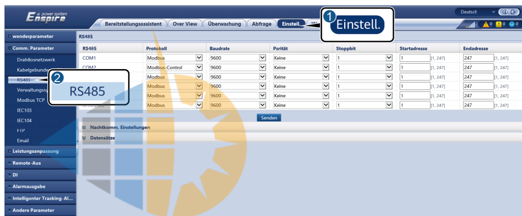
Abbildung 6-93 Einstellen der RS485-Parameter
