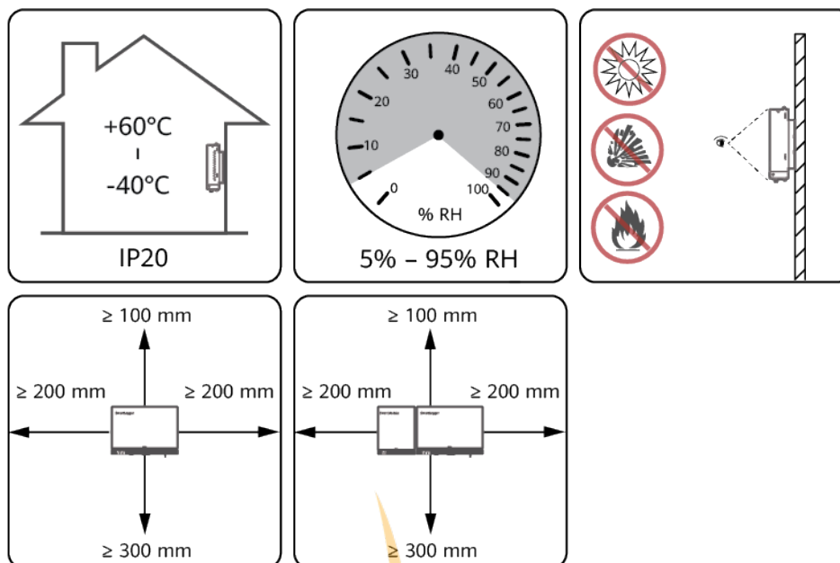
Abbildung 3-1 Einbauposition
