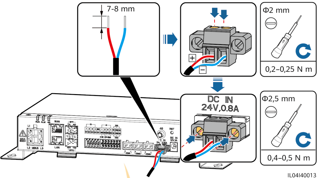
Abbildung 4-13 Anschließen des Eingangsstromkabels
