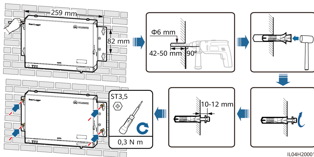
Abbildung 3-2 Wandmontage
