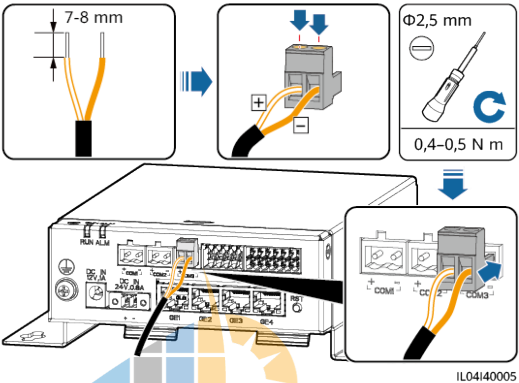
Abbildung 4-17 Anschließen eines RS485-Kommunikationskabels
