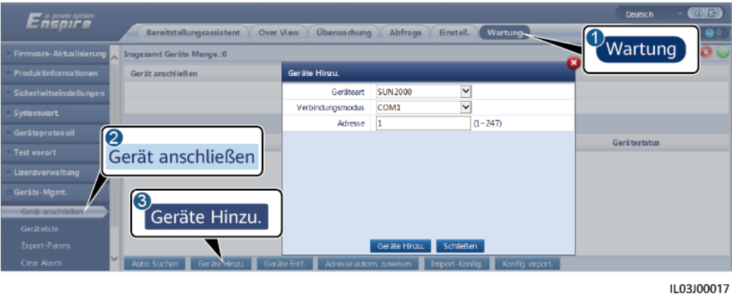
Abbildung 6-54 Einstellen von Zugriffsparametern
