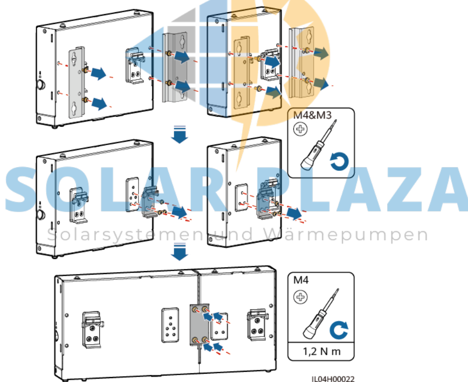
Abbildung 3-7 Verbinden des SmartLoggers mit dem SmartModule mithilfe einer Verbindungsplatte
