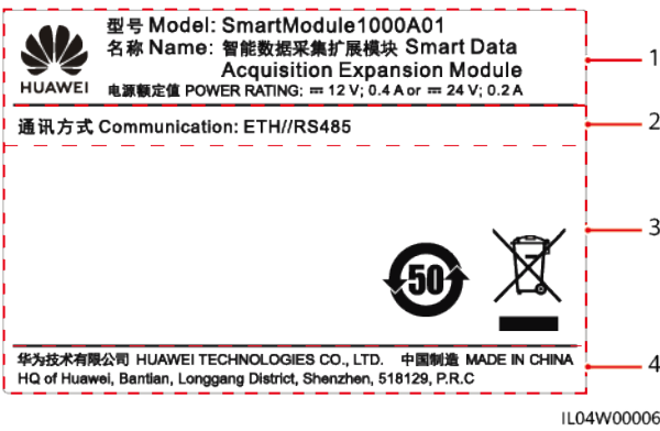
Abbildung 2-10 Typenschild
