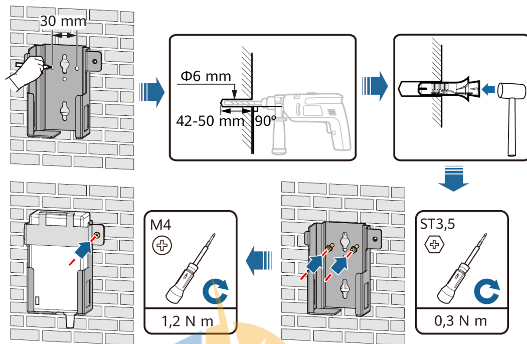
Abbildung 3-10 Wandmontage (Modus 2)
