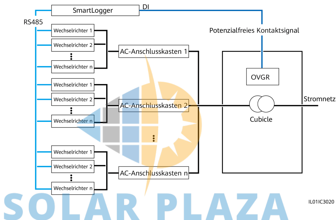
Abbildung 6-88 Vernetzung
