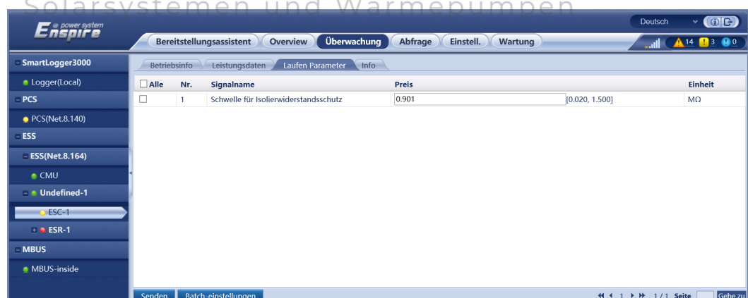
Abbildung 6-49 Festlegen der Betriebsparameter
