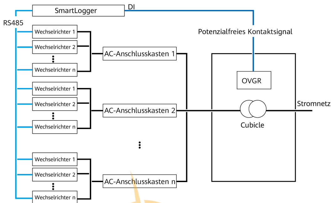
Abbildung 6-89 Vernetzung
