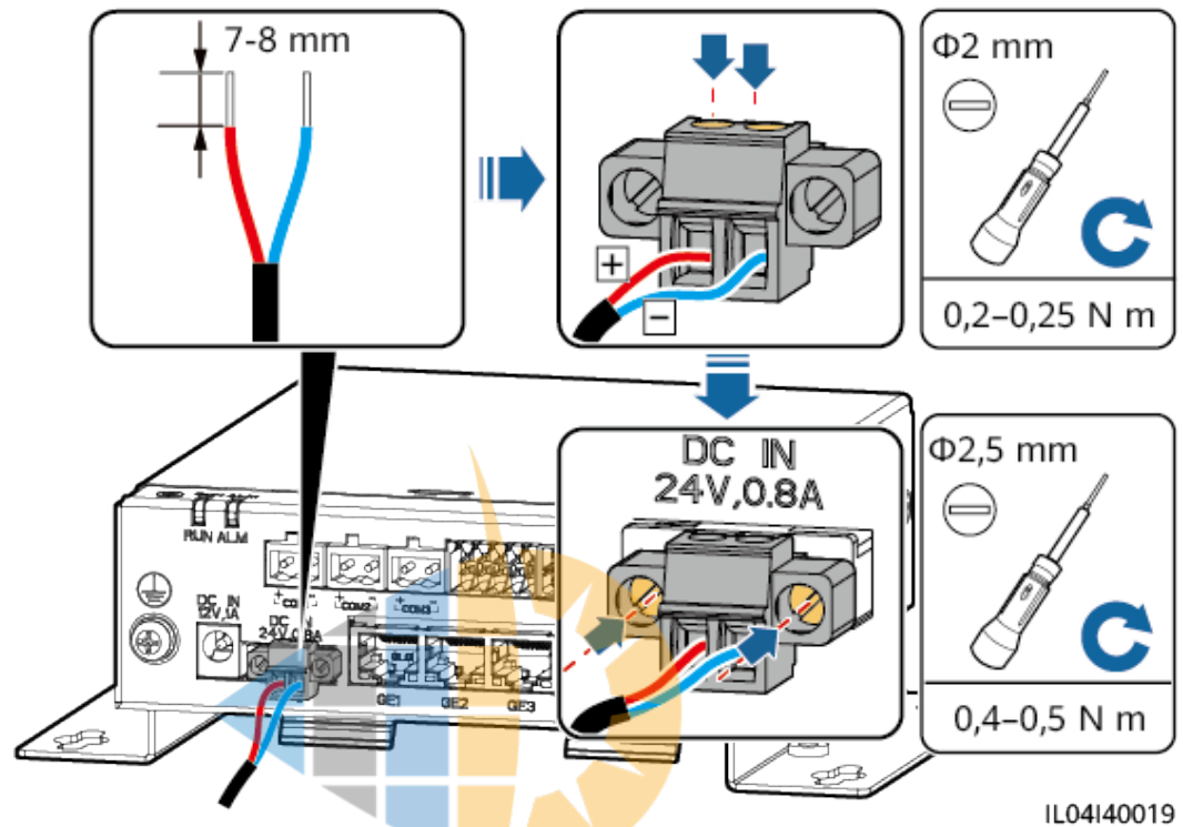
Abbildung 4-24 Anschließen des Eingangsstromkabels
