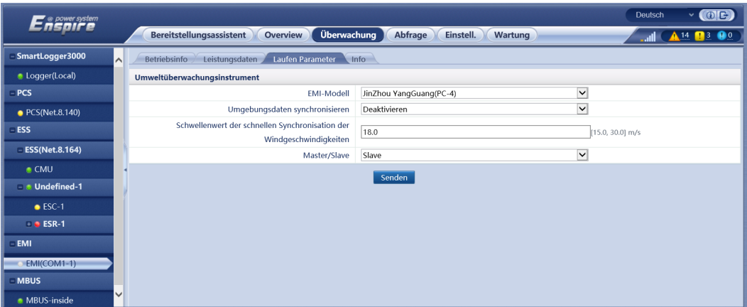
Abbildung 6-63 Einstellen von Betriebsparametern
