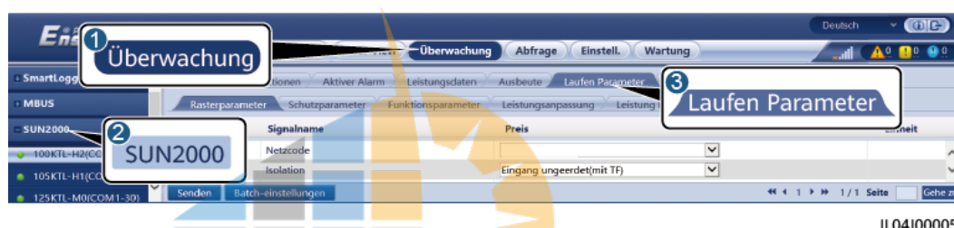
Abbildung 6-41 Einstellen von Betriebsparametern
