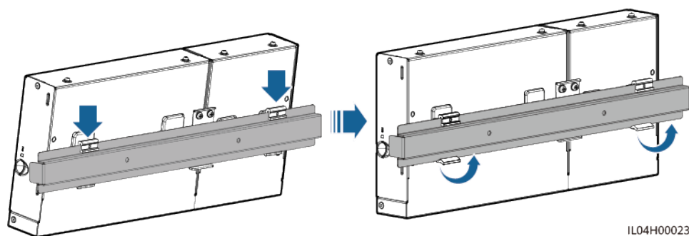
Abbildung 3-8 Tragschienenmontage
