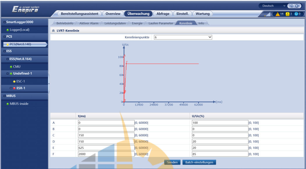
Abbildung 6-46 Kennlinie
