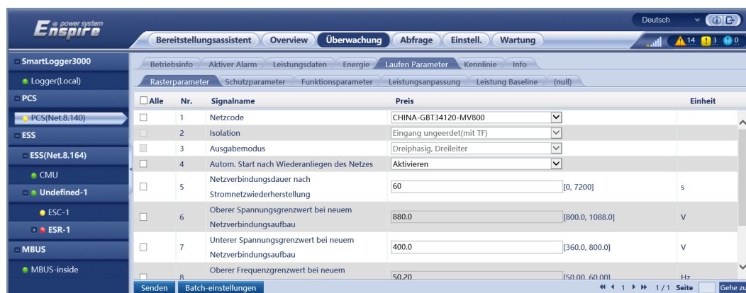
Abbildung 6-45 Festlegen der Betriebsparameter
