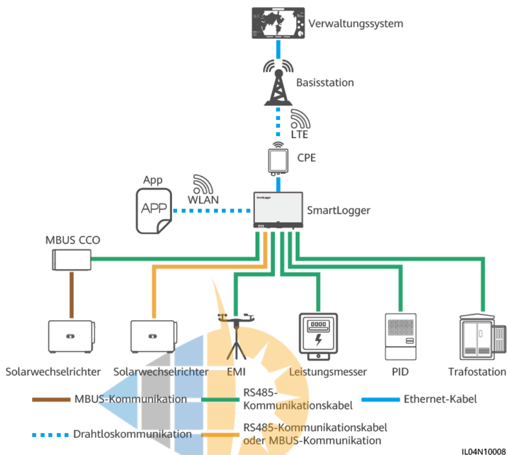
Abbildung 2-6 Dediziertes LTE-Netz
