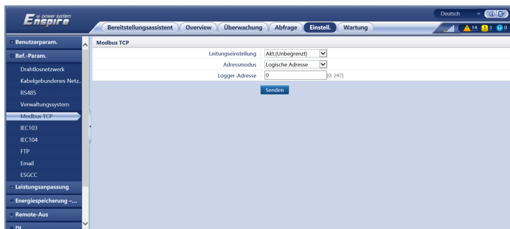
Abbildung 6-31 Einstellen von Modbus-TCP-Parametern
