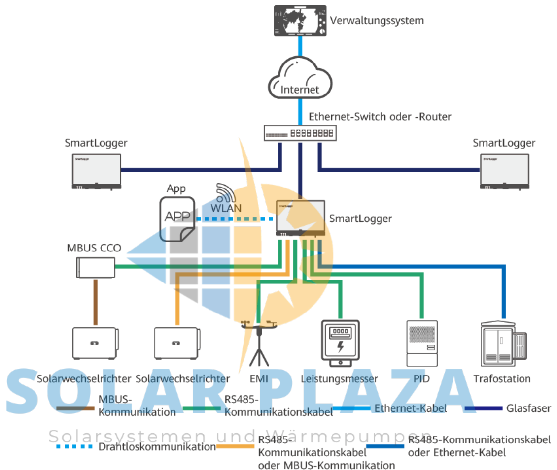
Abbildung 2-4 LWL- oder Ethernet-Sternnetzwerk
