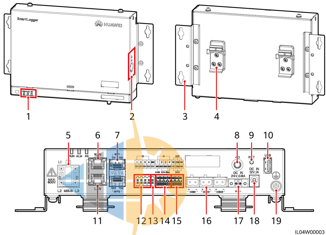
Abbildung 2-7 SmartLogger
