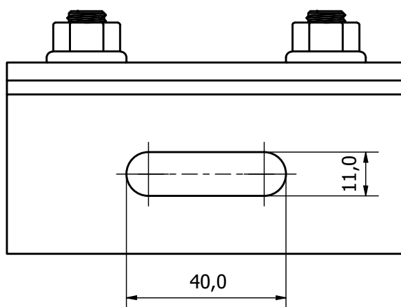
Abb.1 Abmessungen der Konsole K-24-Z
