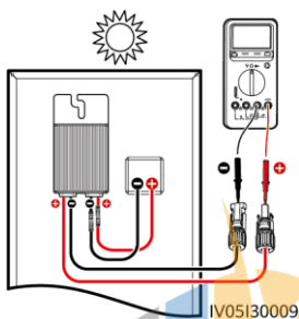
Aansluitdoos van de PV-module
