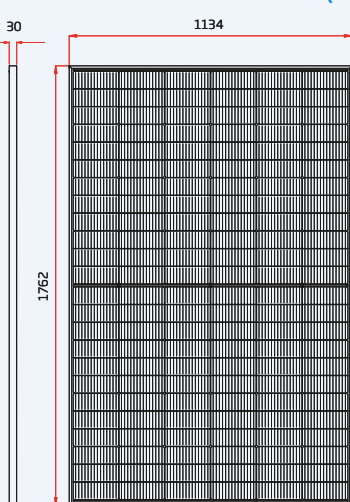
Frontansicht
