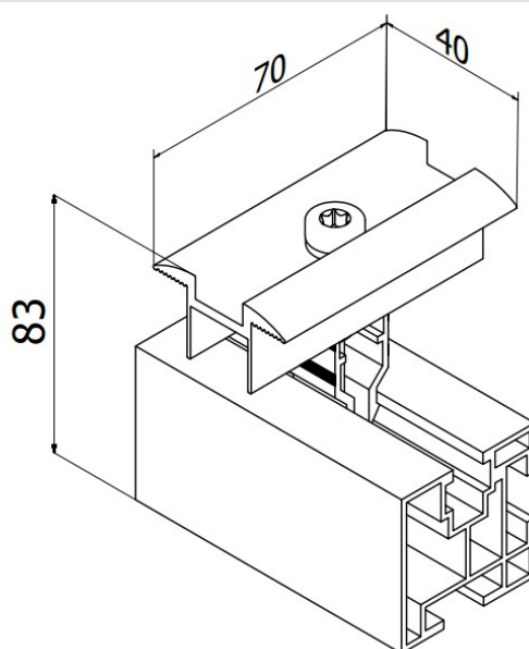
Abb. 1 Abmessungen des Elements K-05-R
