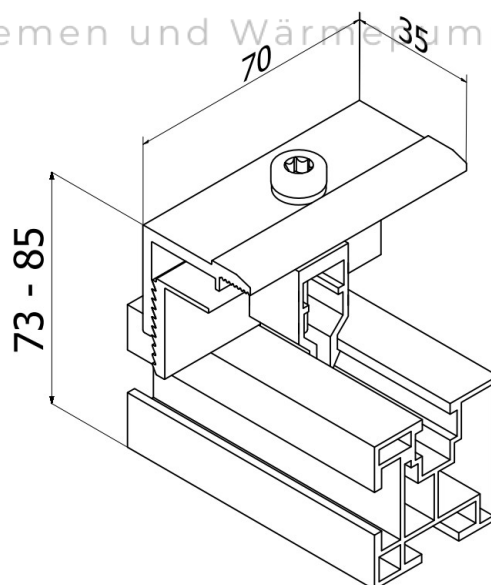
Abb. 2 Abmessungen des Elements K-06-R
