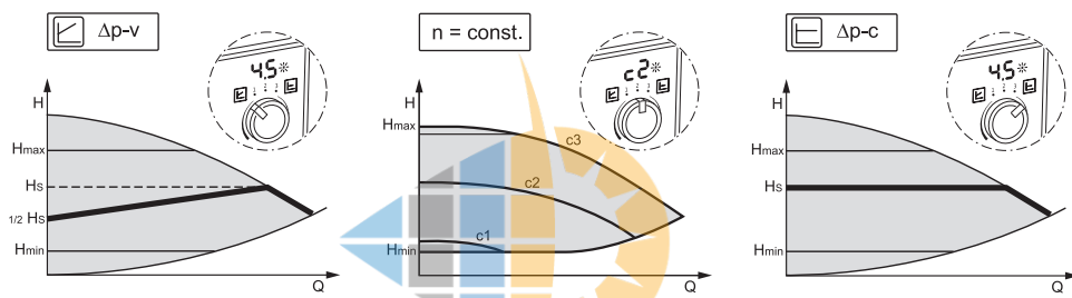
Fig. 4: Betriebsmodus wählen
