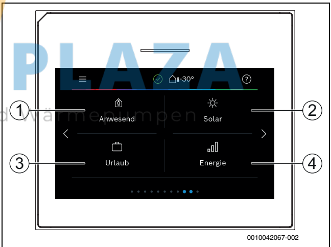
Bild 10 Bedienfeld
