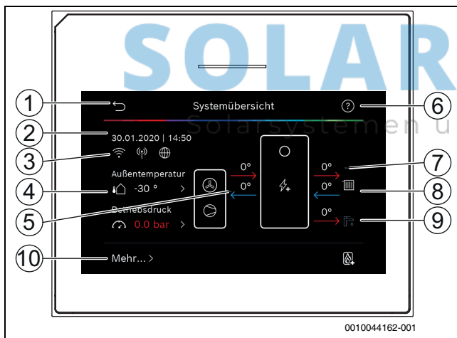
Bild 12 Systemübersicht
