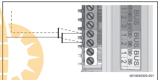
Bild 27 EMS-Anschluss
