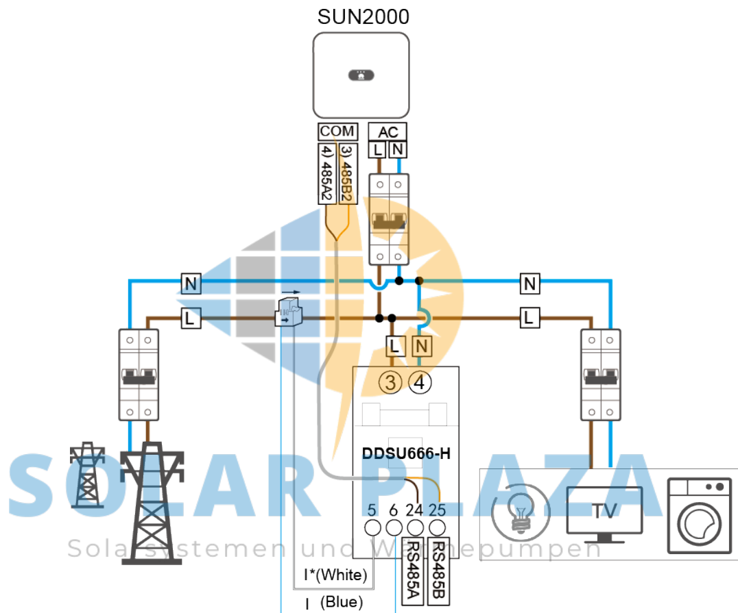
Abbildung 5-28 Anschließen von Kabeln an den Leistungsmesser DDSU666-H
