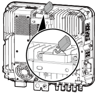
Abbildung 4-10 Installieren eines Diebstahlschutz-Schlusses
