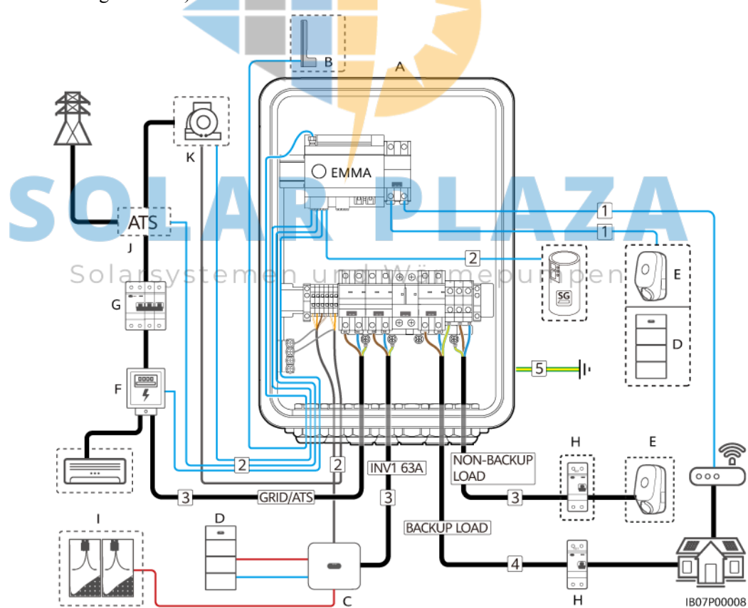
Abbildung 5-1 Kabelverbindungen (gestrichelte Kästchen stehen für optionale Konfigurationen)
