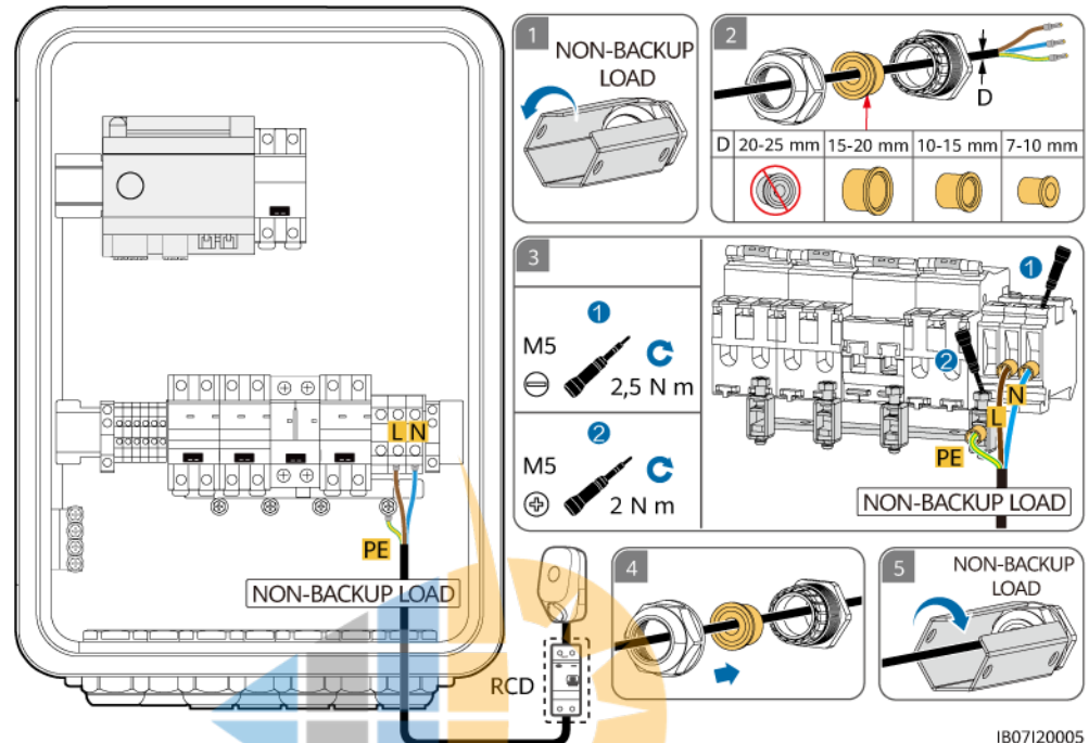
Abbildung 5-17 Anschließen des Ausgangsstromkabels für Nicht-Backup-Lasten (die Komponente im gestrichelten Kästchen ist optional)
