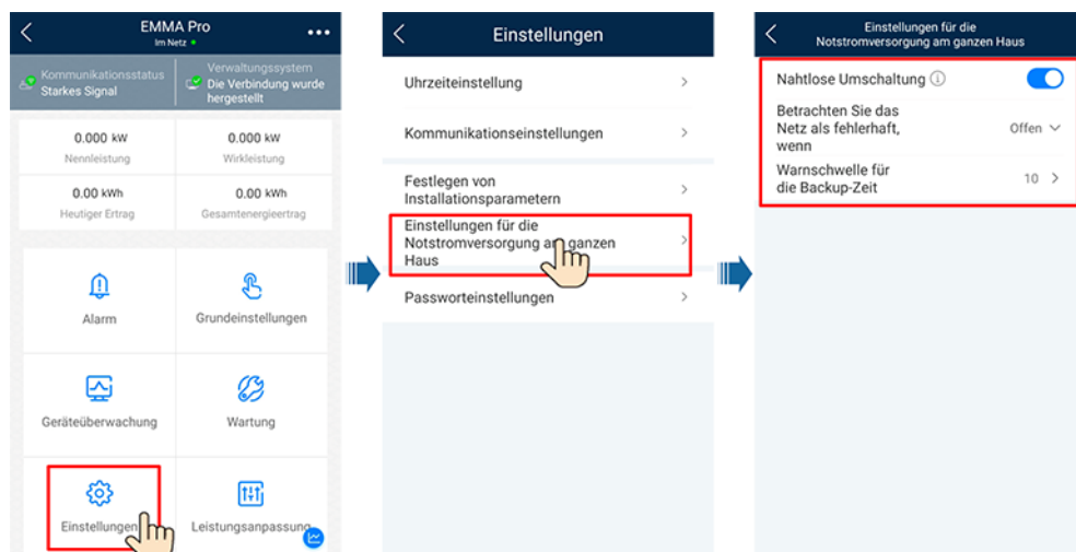
Abbildung 6-4 Einstellungen für die Notstromversorgung am ganzen Haus
