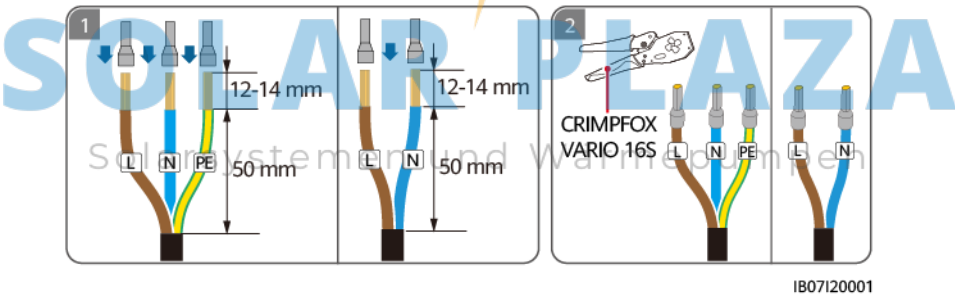
Abbildung 5-10 Crimpen der AC-Kabelendverschlüsse
