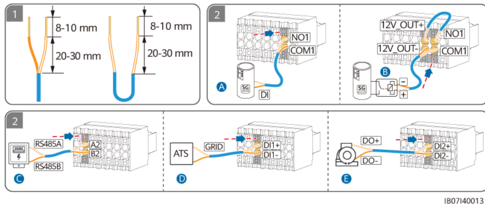
Abbildung 5-22 Anschluss des Signalkabels an die 14-polige Klemme
