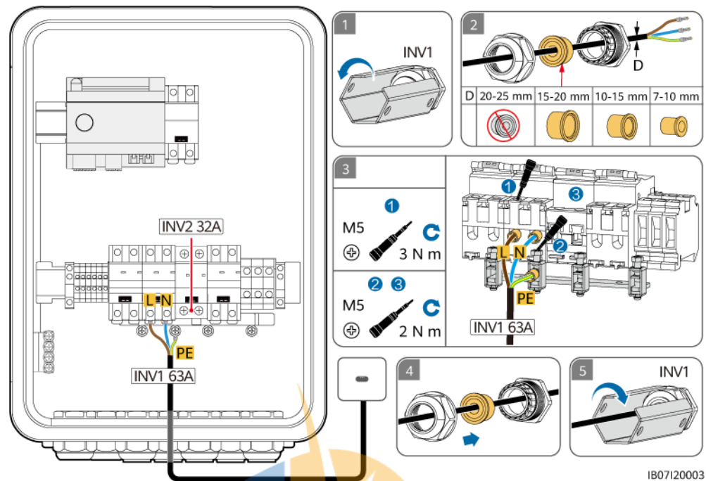
Abbildung 5-11 Anschließen des AC-Eingangsstromkabels des Wechselrichters
