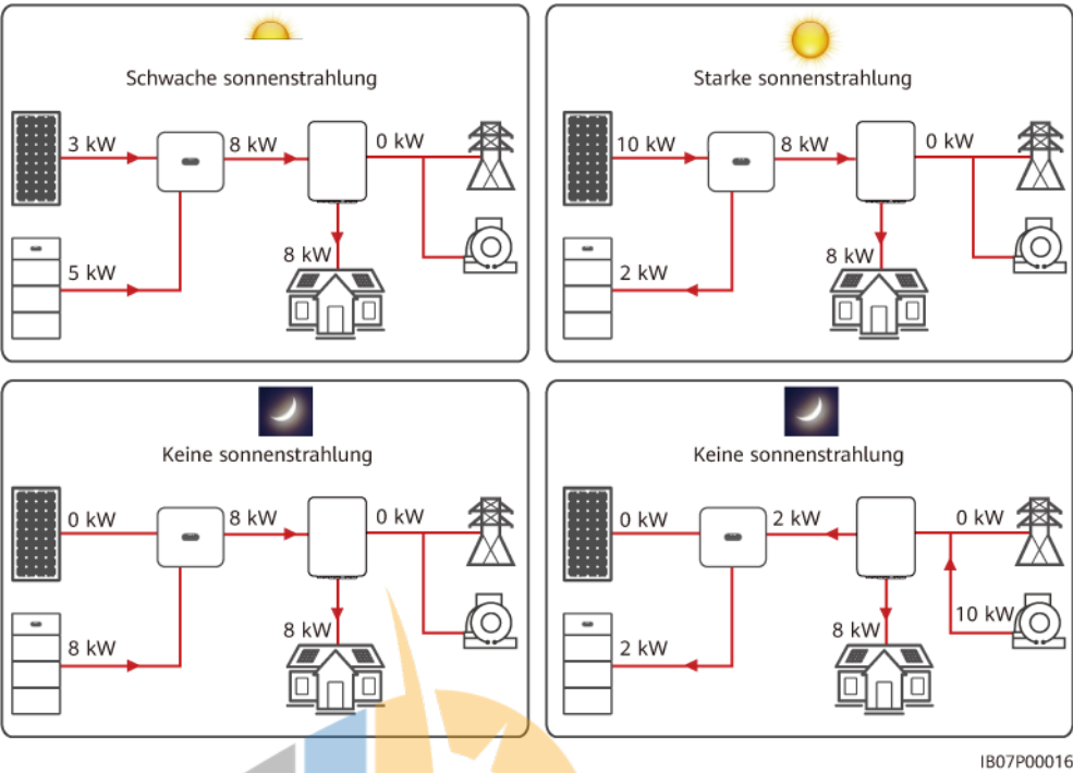
Abbildung 2-6 Darstellung der maximalen Leistung im netzentkoppelten Modus
