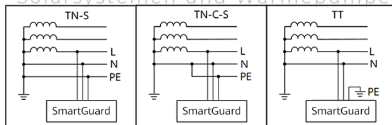
Abbildung 2-7 Erdungssysteme
