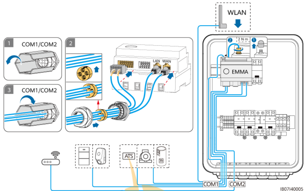
Abbildung 5-25 Anschluss von EMMA-Signalkabeln (gestrichelte Kästchen weisen auf optionale Komponenten hin)
