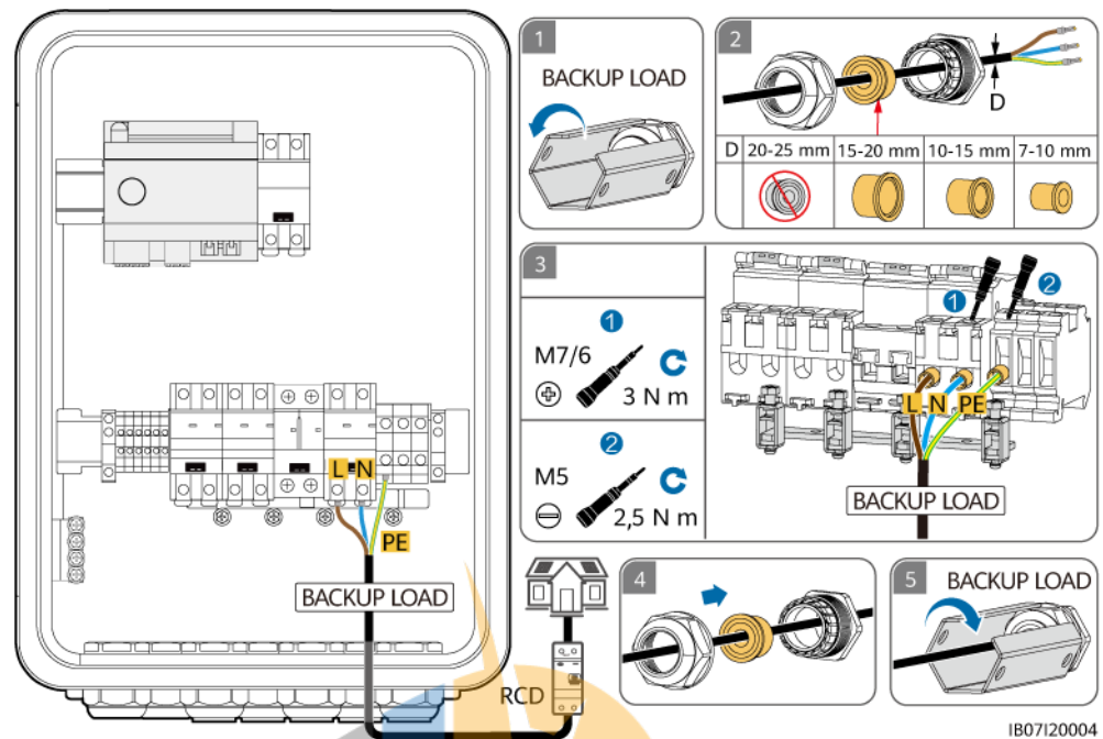
Abbildung 5-14 Anschließen des Ausgangstromkabels der Backup-Last der SmartGuard-63A-S0
