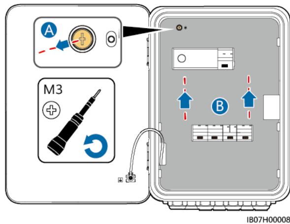
Abbildung 5-6 Öffnen des Deckels des Wartungsfachs
