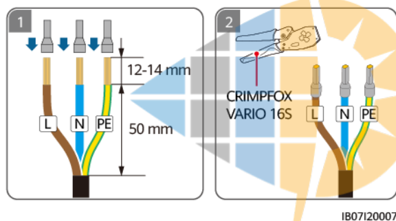
Abbildung 5-12 Crimpen der AC-Kabelendverschlüsse des SmartGuard-63A-S0
