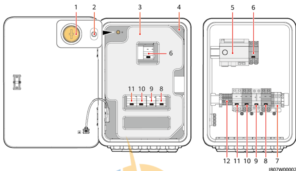
Abbildung 2-9 Wartungsfach und Verdrahtungsklemmen
