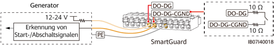
Abbildung E-1 Steuersignal des Generators
