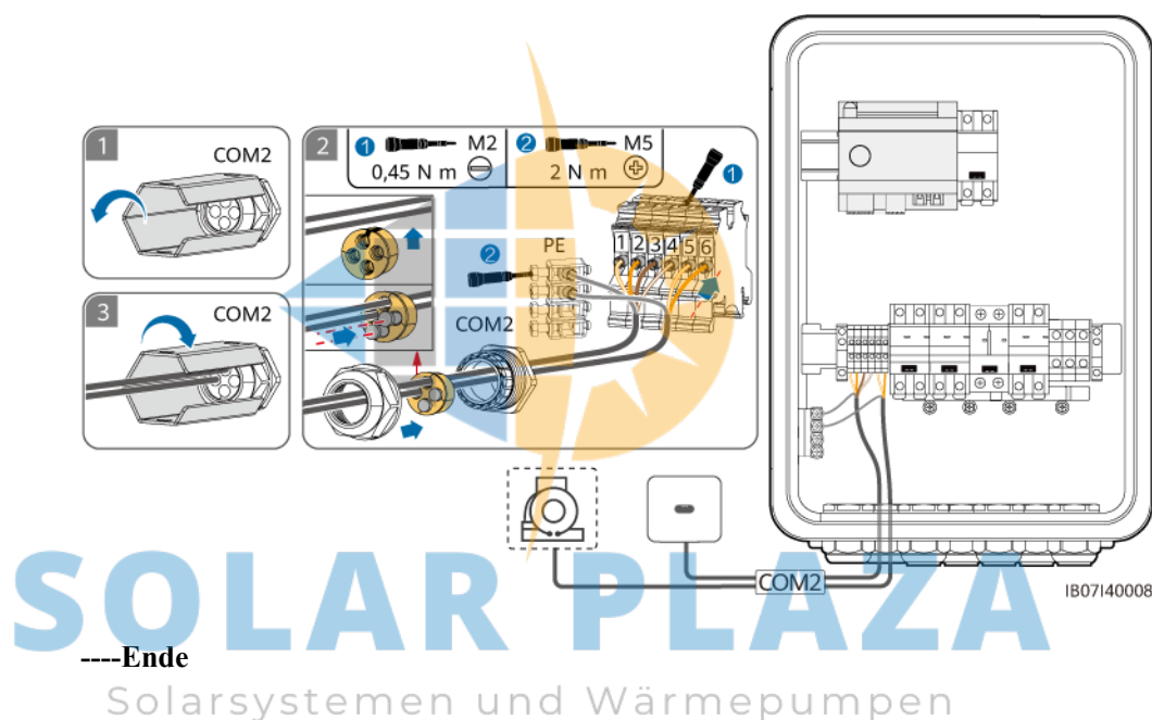
Abbildung 5-19 Anschließen des Signalkabels des SmartGuard (das gestrichelte Kästchen zeigt eine optionale Komponente an)
