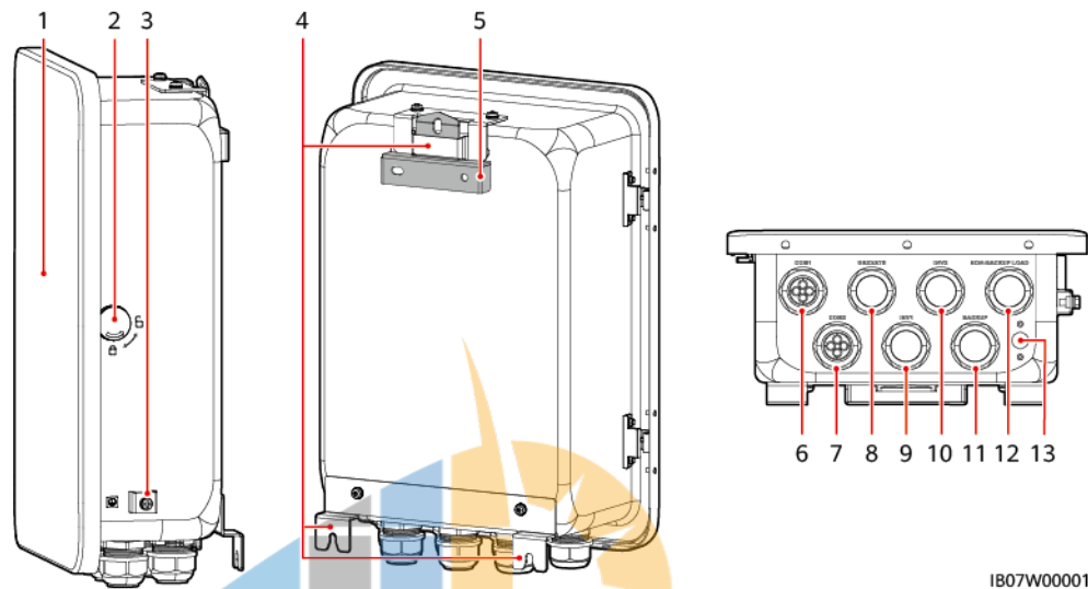
Abbildung 2-8 Aussehen und Anschlüsse
