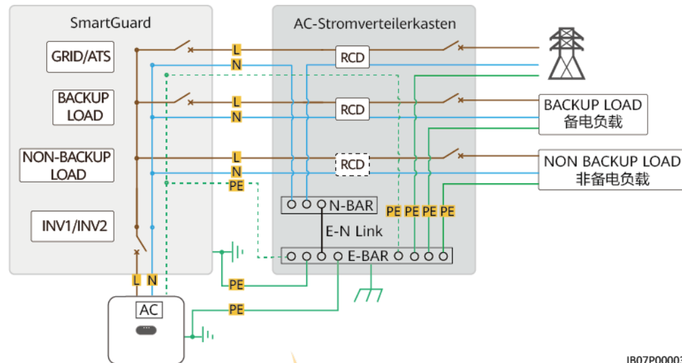
Abbildung 2-3 SmartGuard-63A-AUS0 Schaltplan für Wohngebäude (gestrichelte Linien stehen für optionale Kabelanschlüsse)
