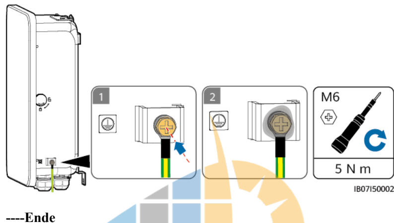
Abbildung 5-4 Anschließen des PE-Kabels
