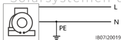
Abbildung 5-7 Generator-Nullleiter-Erdung
