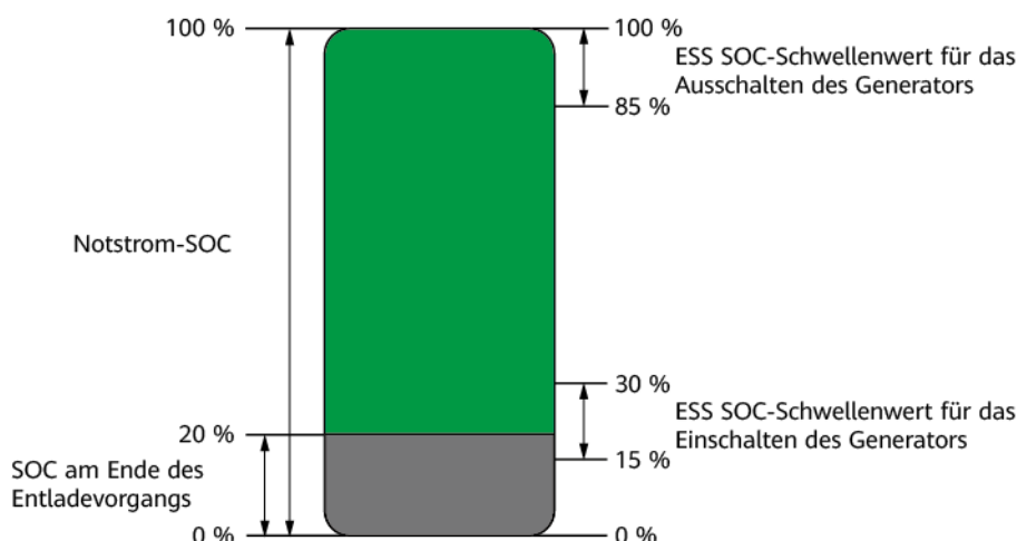
Abbildung 6-10 Batterie-SOC
