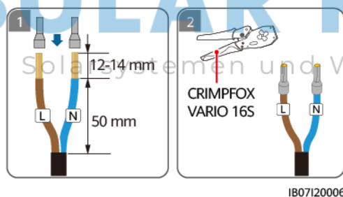
Abbildung 5-13 Crimpen der AC-Kabelendverschlüsse des SmartGuard-63A-AUS0
