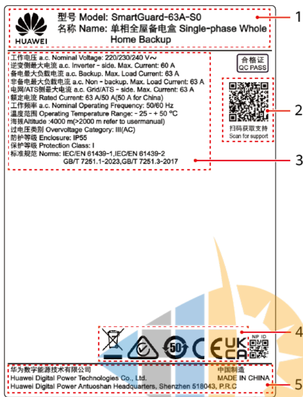
Abbildung 2-12 Typenschild (am Beispiel von SmartGuard-63A-S0)
