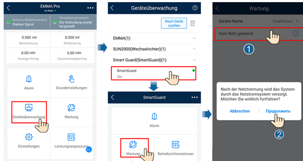
Abbildung 6-11 Einstellen des Umschaltens zwischen netzgekoppeltem und netzentkoppeltem Modus
