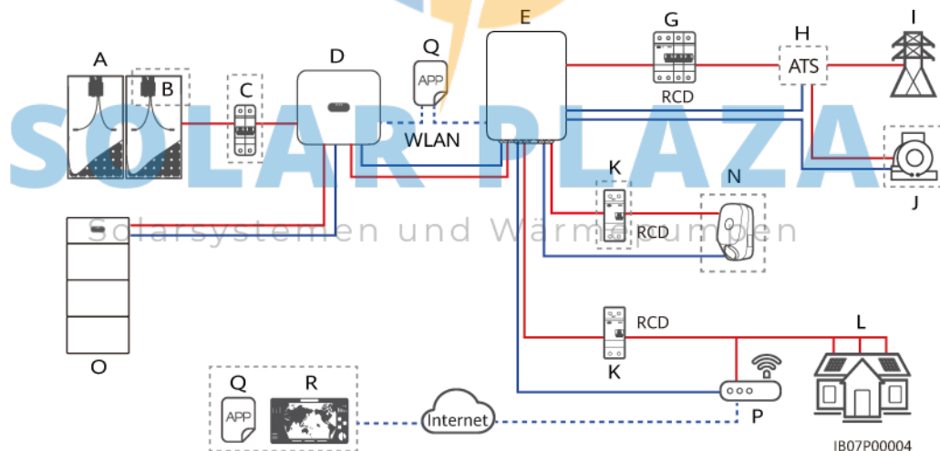
Abbildung 2-4 Vernetzung aller Lasten, die an die SmartGuard angeschlossen sind (gestrichelte Kästchen weisen auf optionale Komponenten hin)
