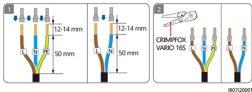
Abbildung 5-16 Crimpen der AC-Kabelendverschlüsse
