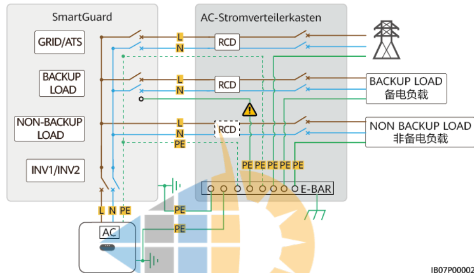
Abbildung 2-2 SmartGuard-63A-S0 Schaltplan für Wohngebäude (gestrichelte Linien stehen für optionale Kabelanschlüsse)
