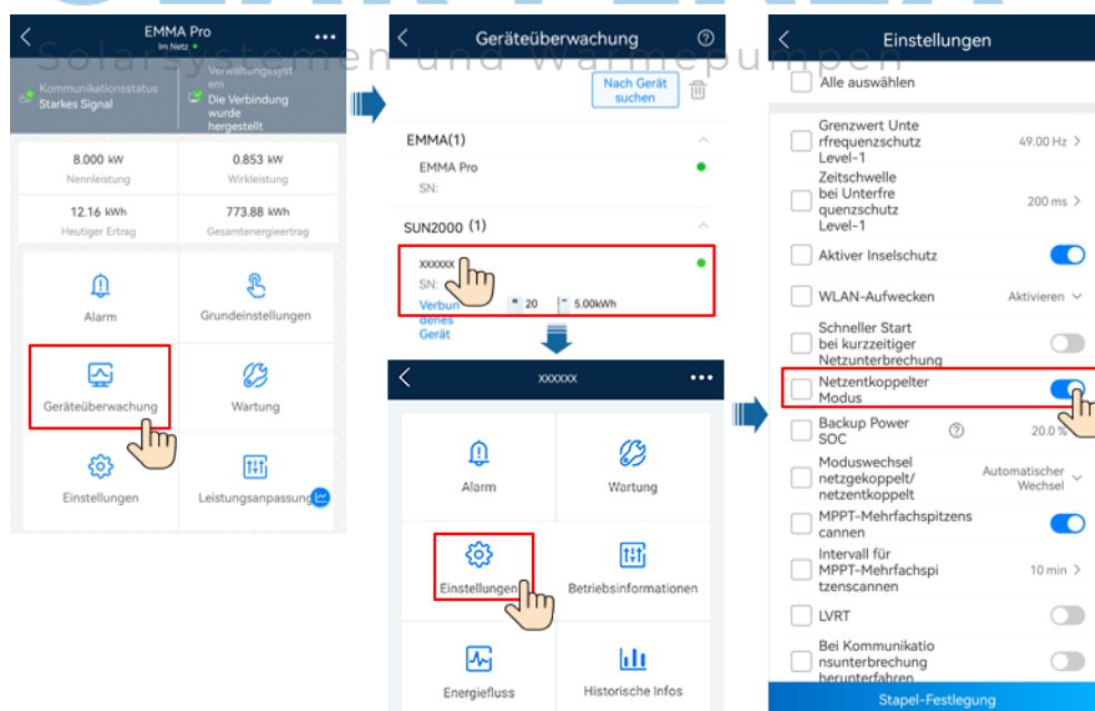
Abbildung 6-5 Einstellen des netzentkoppelten Modus
