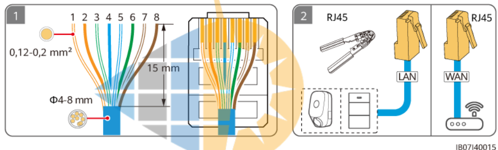
Abbildung 5-24 FE-Kommunikationskabel (gestrichelte Kästchen weisen auf optionale Komponenten hin)
