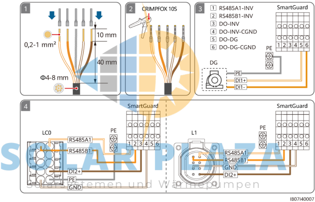
Abbildung 5-18 Crimpen der Kabelendverschlüsse des Signalkabels (das gestrichelte Kästchen zeigt eine optionale Komponente an)
