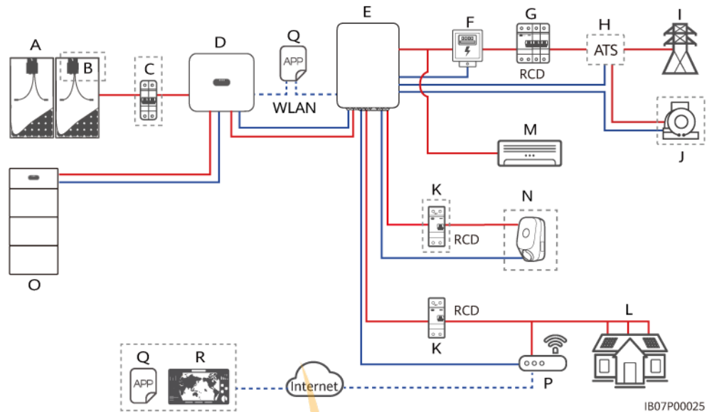
Abbildung 2-5 Vernetzung einiger Lasten, die an die SmartGuard angeschlossen sind (gestrichelte Kästchen weisen auf optionale Komponenten hin)
