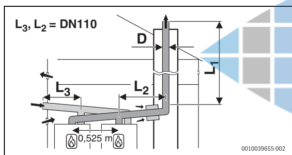
Bild 26 C 53
