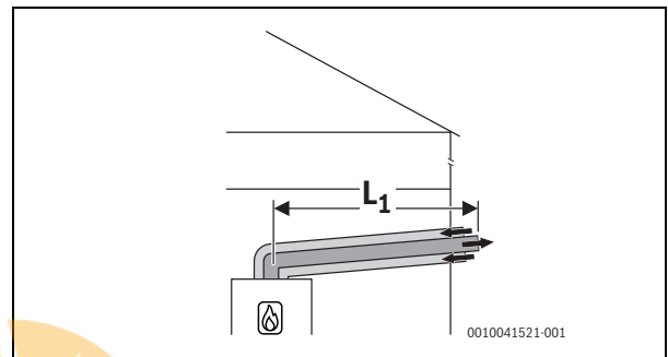
Bild 8 C 13(x)
