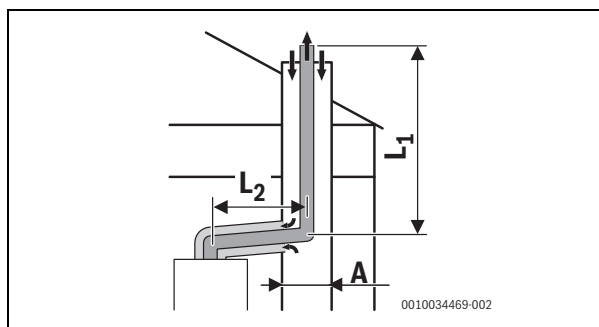
Bild 17 C 93(x)
