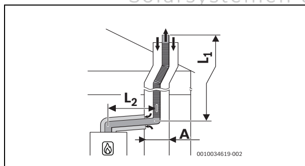
Bild 18 C 93x
