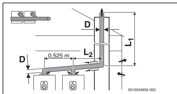
Bild 24 B 23p /B 53p
