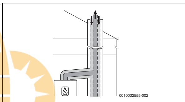
Bild 11 C 43(x)
