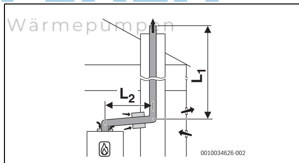
Bild 19 B 53p
