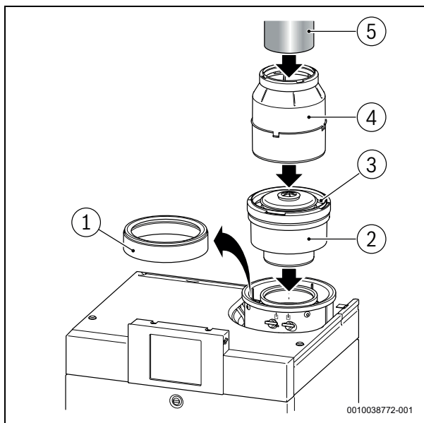
Bild 5 Montieren des externen Abgasrückschlagventils
