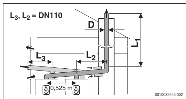
Bild 27 C 53
