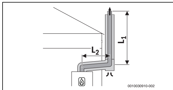
Bild 15 C 53x
