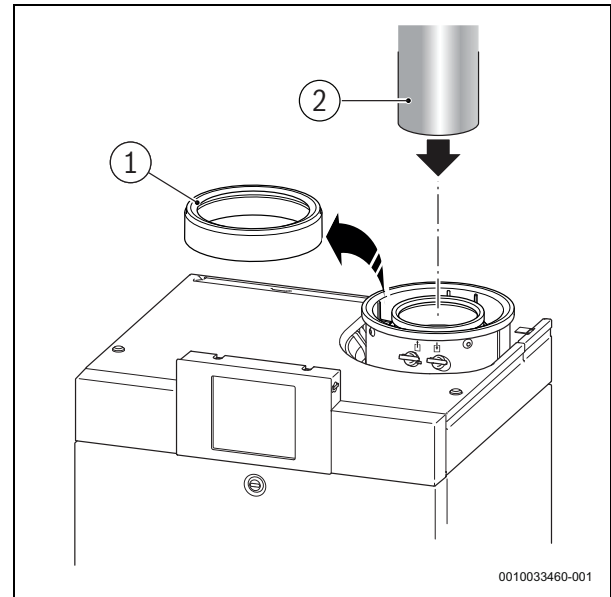
Bild 4 Einzelrohranschluss (raumluftabhängig)
