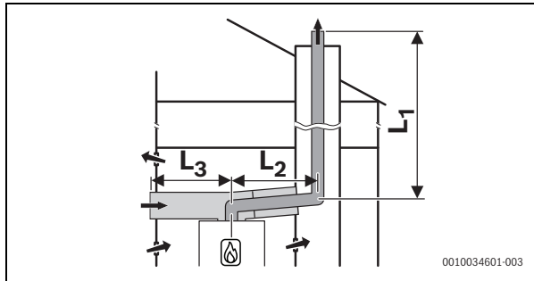
Bild 12 C_{53(x)}
