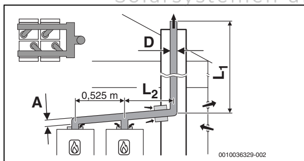
Bild 25 B 23p /B 53p
