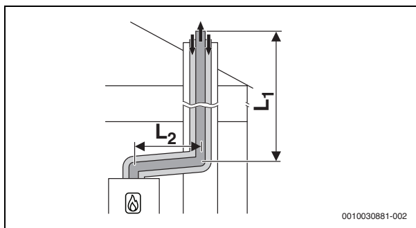
Bild 9 C 33(x)
