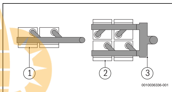
Bild 21 Draufsicht Kaskadenaufstellung
