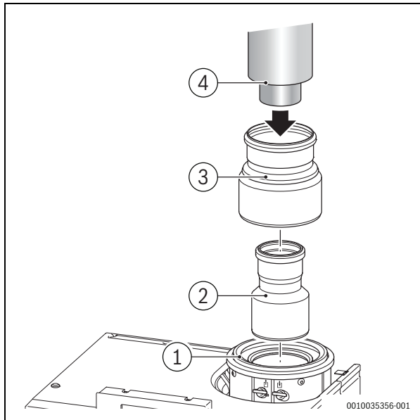
Bild 3 Montieren des Abgasadapters Ø 80/125
