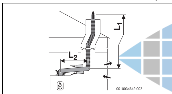
Bild 20 B 53p
