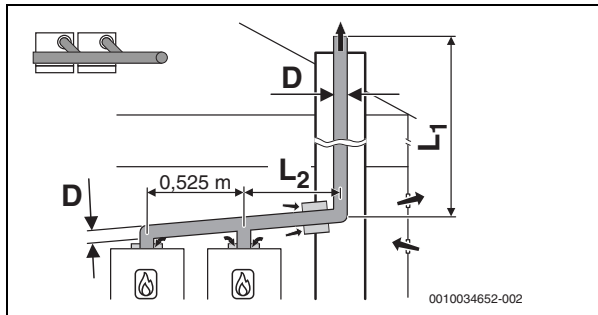
Bild 22 B 23p /B 53p
