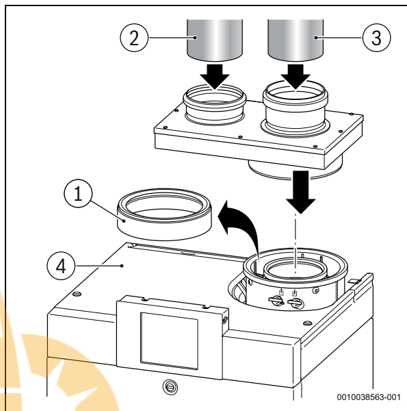
Bild 2 Montieren des Abgasadapters Ø 110-110
