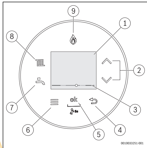
Bild 6 Bedienfeld
