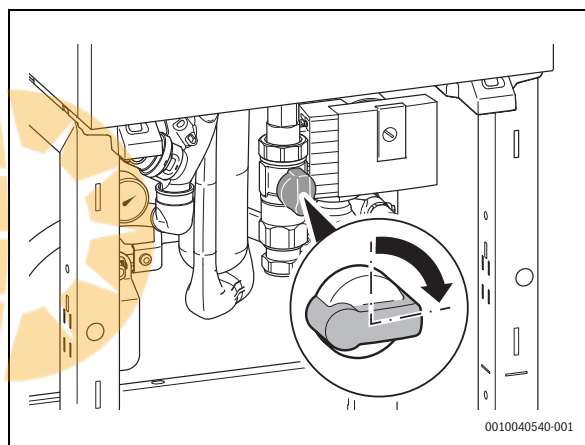
Bild 3 Schließen des Gashahns
