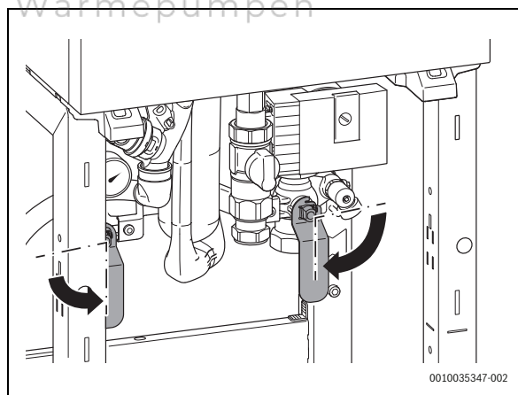
Bild 4 Öffnen der Serviceabsperrrventile
