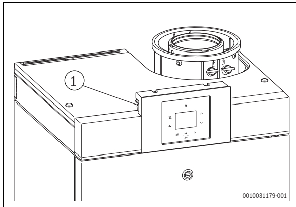
Bild 5 Schalter Ein/Aus
