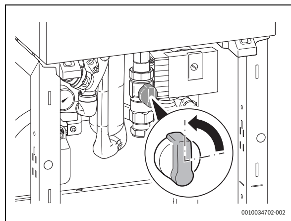
Bild 2 Öffnen des Gashahns
