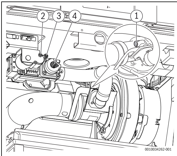
Bild 32 Übersicht Messstutzen und Stellschrauben ≤ 70 kW
