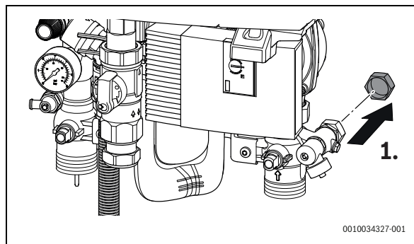
Bild 20 Anschließen eines Ausdehnungsgefäßes
