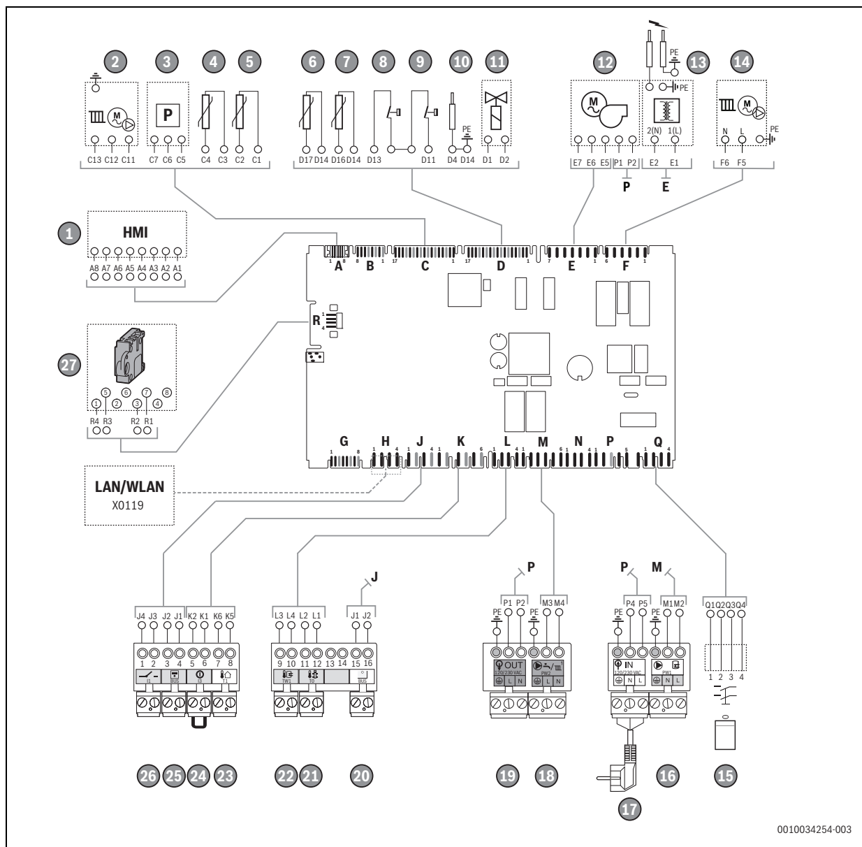
Bild 50 Schaltplan
