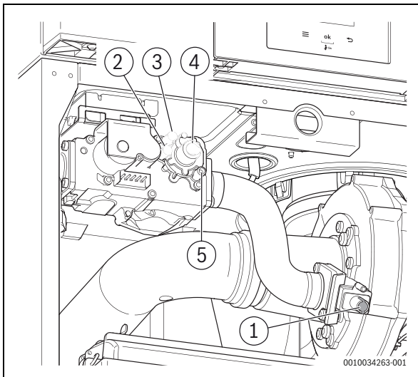
Bild 33 Übersicht Messstutzen und Stellschrauben ≥ 85 kW
