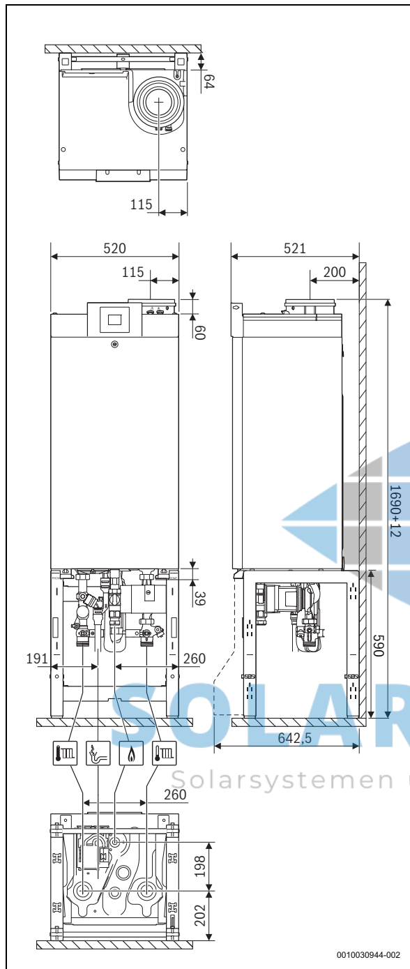
Bild 2 Abmessungen auf Grundgestell [mm]
