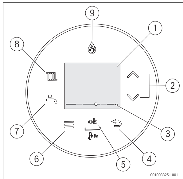
Bild 26 Bedienfeld UI700
