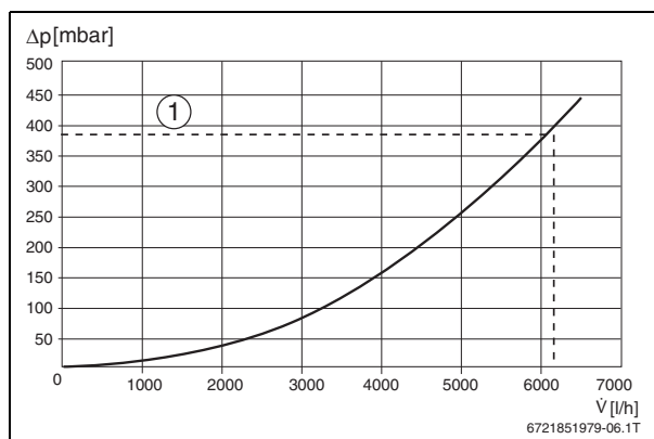
Bild 16 Druckverlust GC7000WP 150
