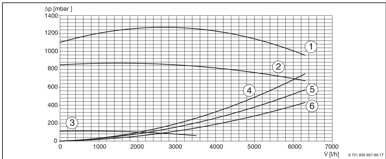
Bild 14 Restförderhöhe GC7000WP 150
