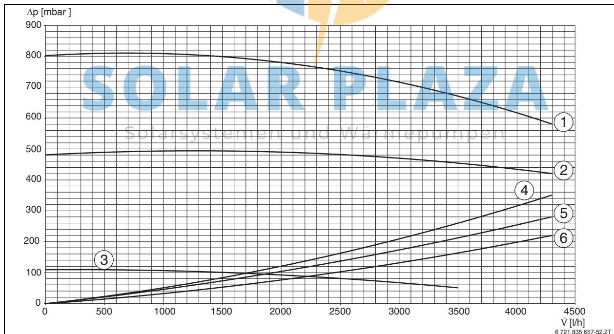
Bild 13 Restförderhöhe GC7000WP 100
