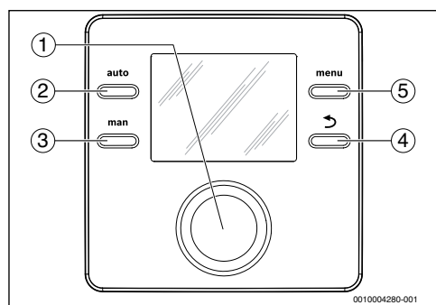
Bild 1 Bedienelemente
