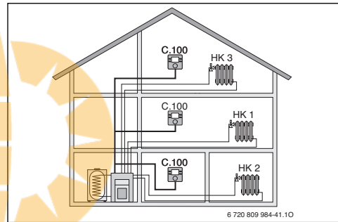
Bild 3 Beispiel für Heizungsanlage mit drei Heizkreisen mit jeweils einer C 100 als Regler (Mehrfamilienhaus)
