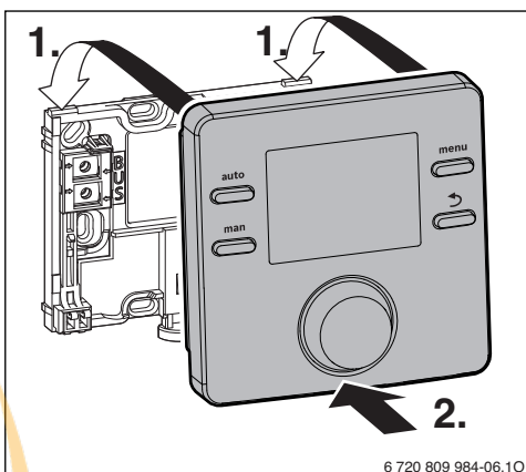
Bild 9 Bedieneinheit einhängen
