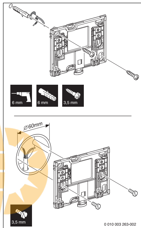
Bild 7 Montage des Sockels
