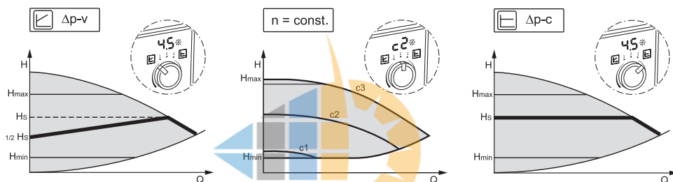
Fig. 4: Betriebsmodus wählen
