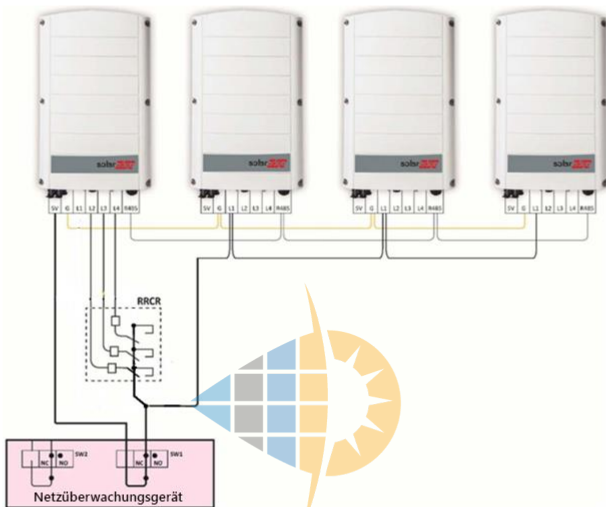
Abbildung 6: RRCR mit drei Relais und AC-Relaissteuerung
