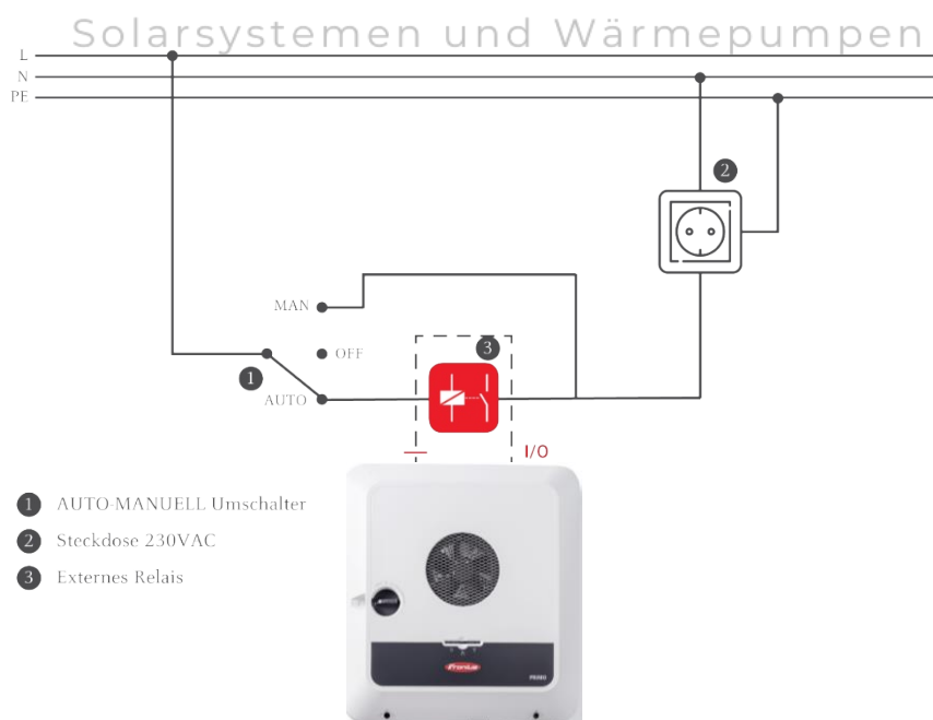
Abbildung 1 – Beispiel Schaltplan
