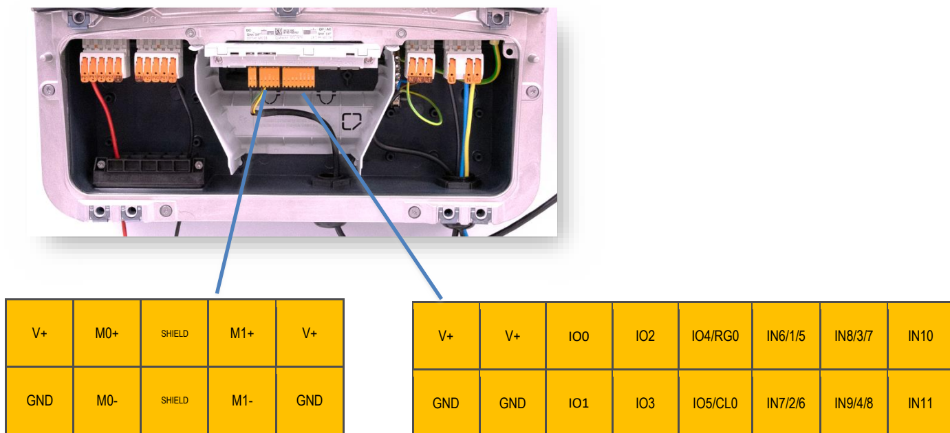
Abbildung 5: 10-poliger Stecker – 2 x Modbus RTU, 16-poliger Stecker digitale Ein-Ausgänge (IO 0-IO 3)
