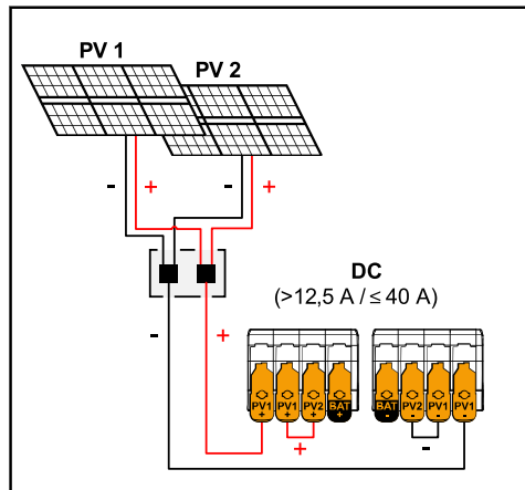
Kombinierte Solarmodul-Stränge mit Summenstrom größer 12,5 A ( I_{dcmax} ).
