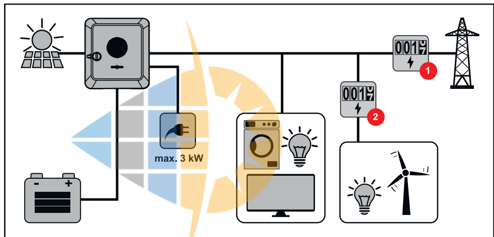
Betriebsmodus - Wechselrichter mit Batterie und mehreren Smart Metern
