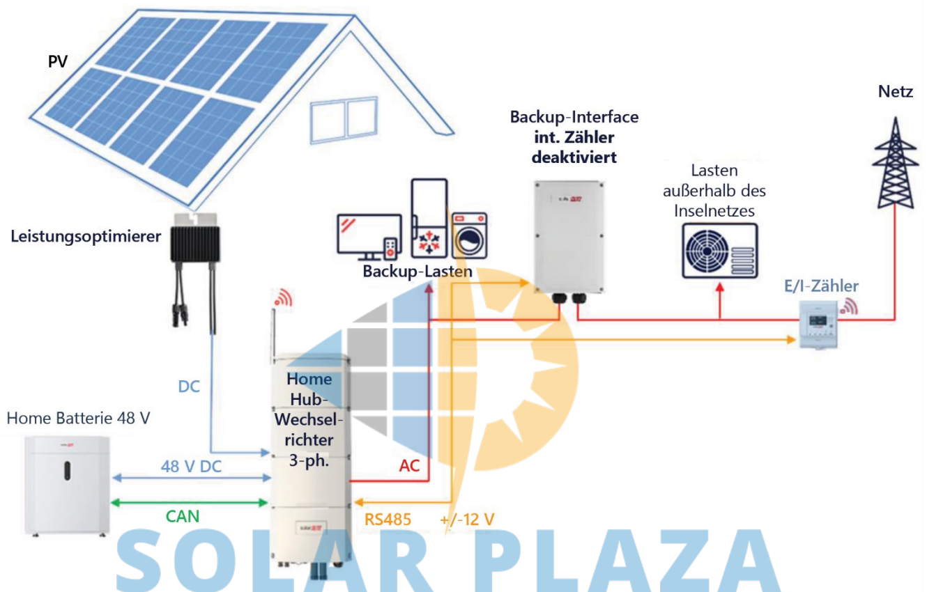
Solarsystemen und Wärmepumpen Abbildung 8 – Ersatzstrom-Installation für partielles Backup
