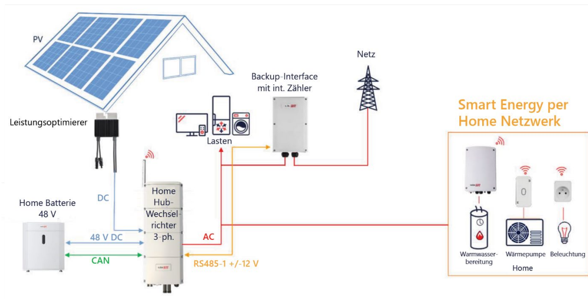
Abbildung 5 – Backup-Installation – einzelner Wechselrichter
