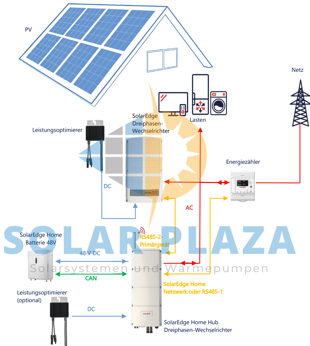
Abbildung 12 – Home Hub Dreiphasen-Wechselrichter, AC-gekoppelt an einem vorhandenen SolarEdge Dreiphasen-Wechselrichter
