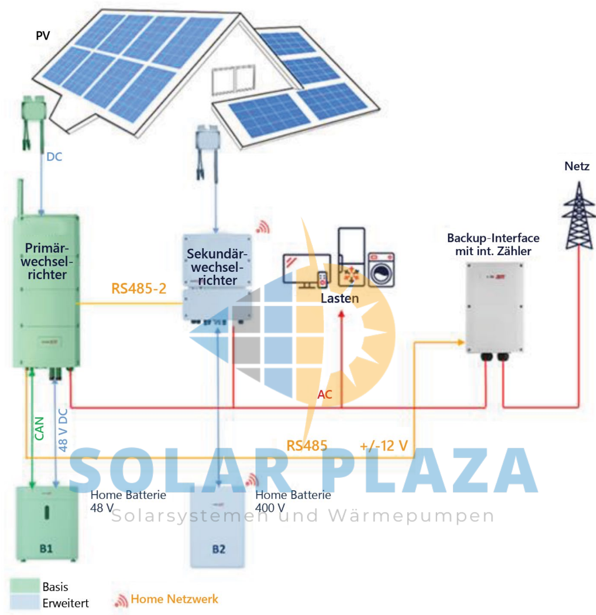
Abbildung 9 – Installation eines Home Hub Dreiphasen-Wechselrichters mit einem StorEdge Einphasen-Wechselrichter
