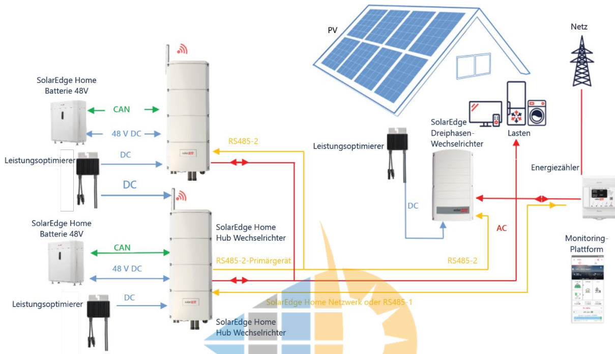
Abbildung 13 – AC-Kopplung – Mehrere SolarEdge Dreiphasen-Wechselrichter
