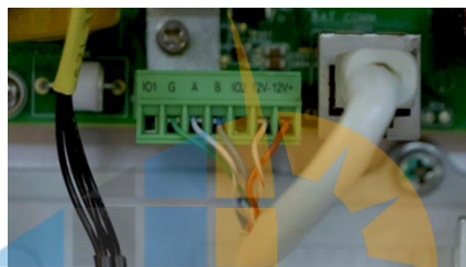
Abbildung 1 – Backup-Interface und Zähleranschlüsse
