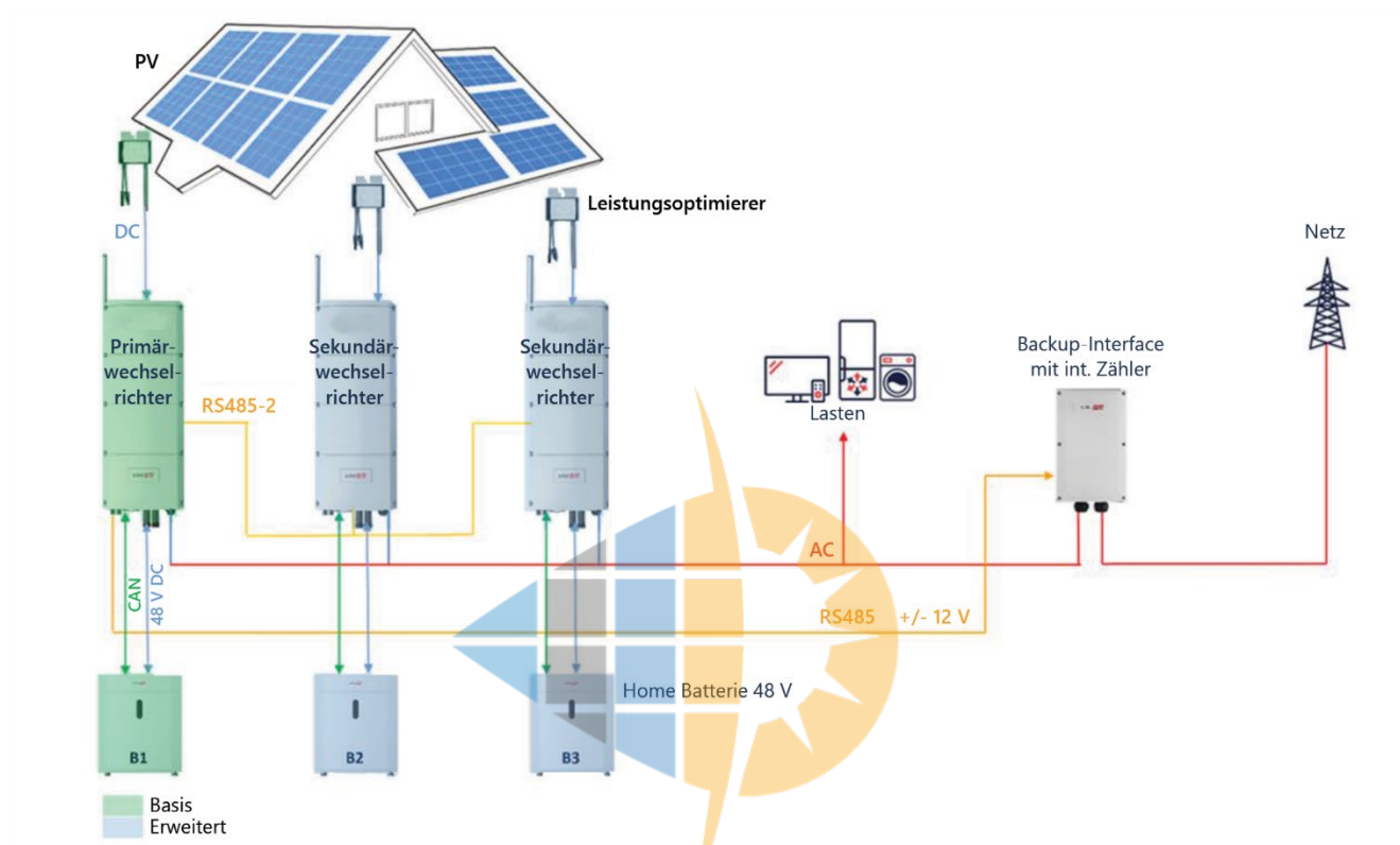
Abbildung 6 – Ersatzstrom-Installation mit mehreren Wechselrichtern, PV-Strängen und Batterien
