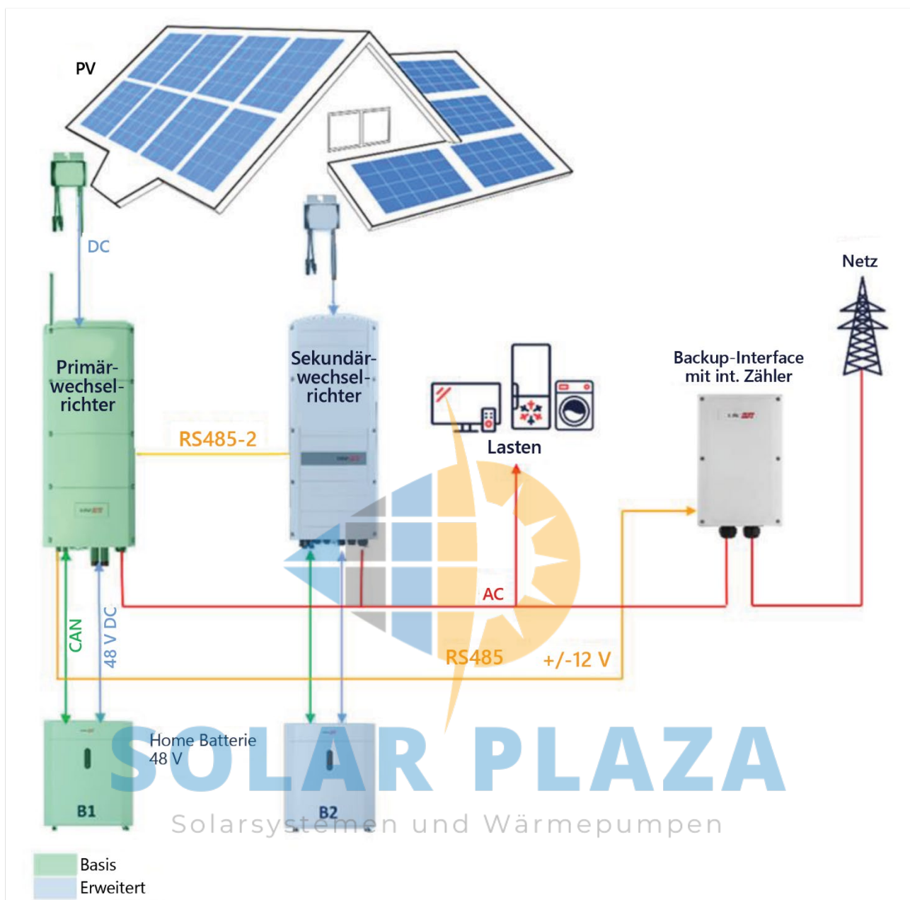
Abbildung 10 – Installation eines Home Hub Dreiphasen-Wechselrichters mit einem StorEdge Dreiphasen-Wechselrichter
