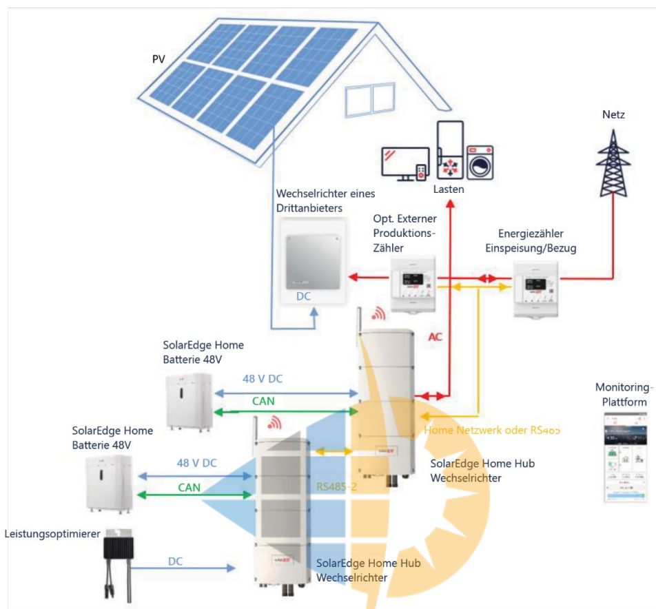
Abbildung 14 – AC-Kopplung mit einer Stromquelle eines Drittanbieters
