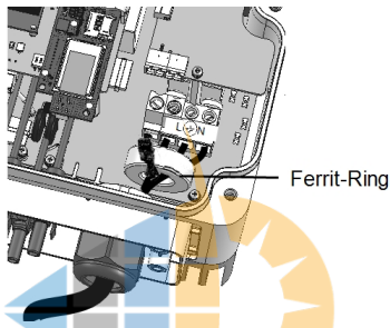
Abbildung 8: AC-Anschluss
