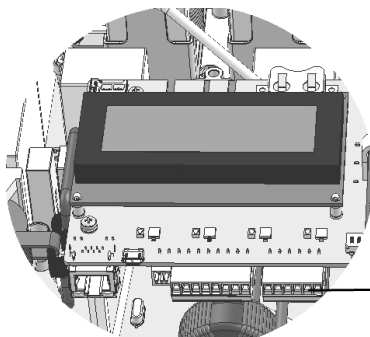
Abbildung 18: Die RS485-Klemmleiste
