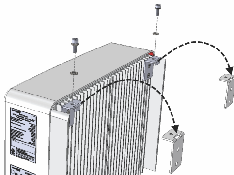
Abbildung 24: Montagehalterungen
