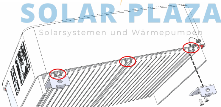
Abbildung 5: Montage der Wechselrichterhalterungen
