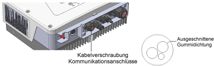
Abbildung 15: Kabelverschraubung und Gummidichtung
