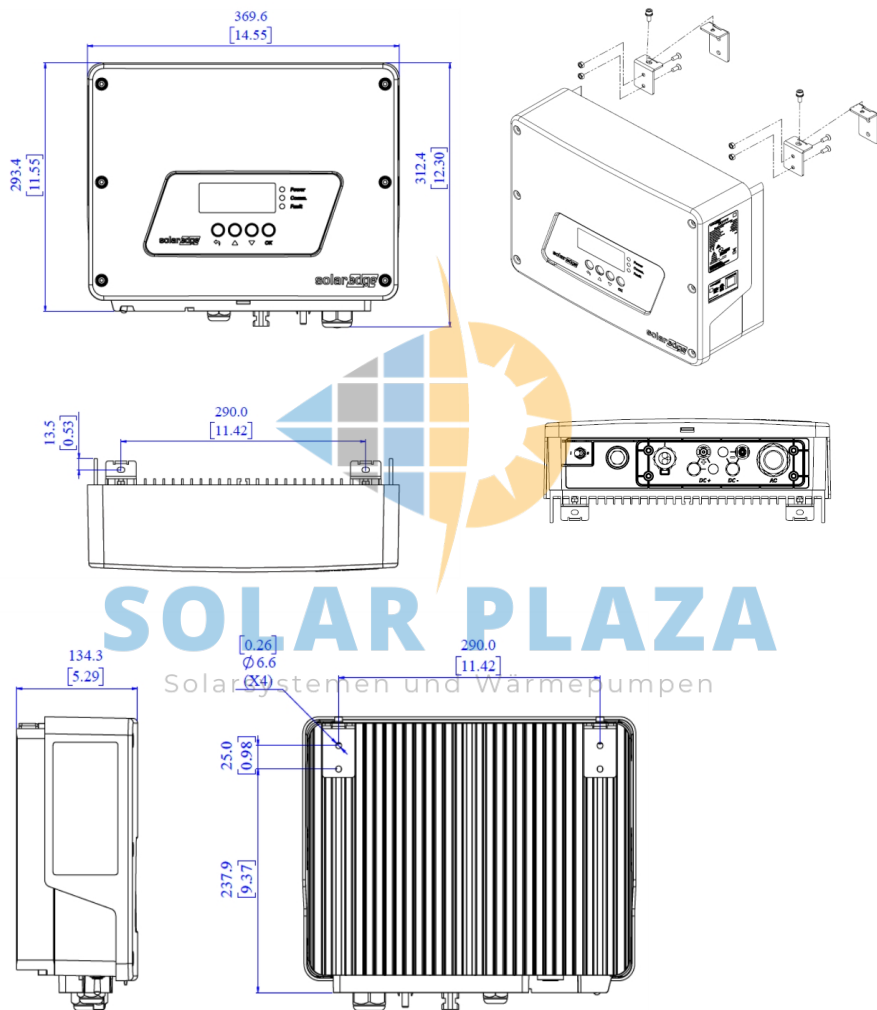
Abbildung 22: HD-Wave-Wechselrichter-Abmessungen
