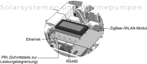
Abbildung 13: Kommunikationskartenanschlüsse
