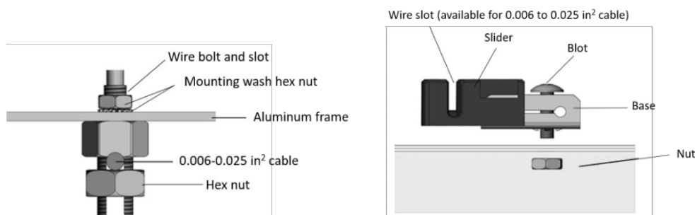
Abbildung 4. Erdungsmethoden für PV-Module (IEC-Norm).
