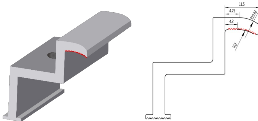
Abbildung 3. A-Oberflächen-Anpassungsklemme
