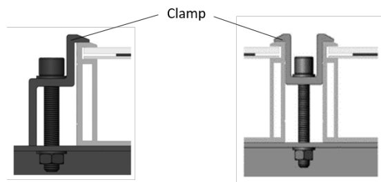
Montage der Endklemme
