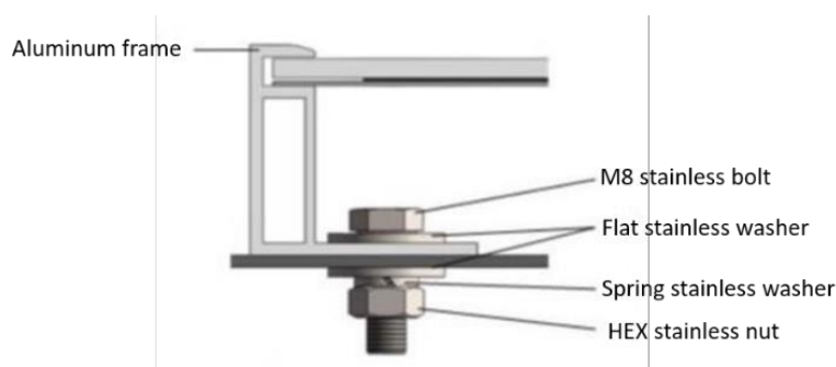
Abbildung 1. PV-Modul, montiert mit Schraubbefestigung.
