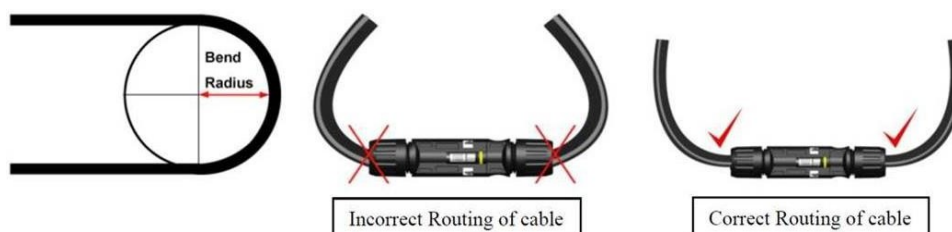
Abbildung 5. Die korrekte Verlegung und der Mindestbiegeradius der Kabel.
