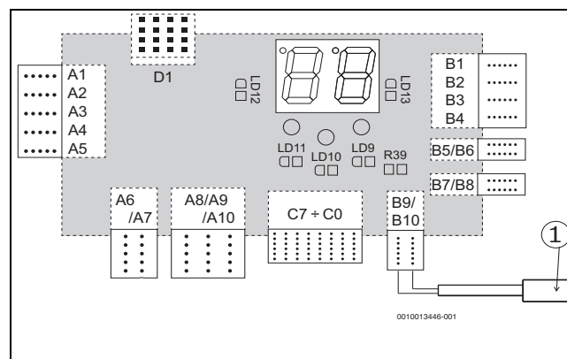
Obr. 10 Pripojenie snímača k svorkám B9/B10
