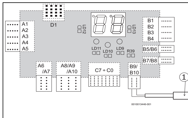
Rys. 17 Podłączenie czujnika do zacisków B9/B10
