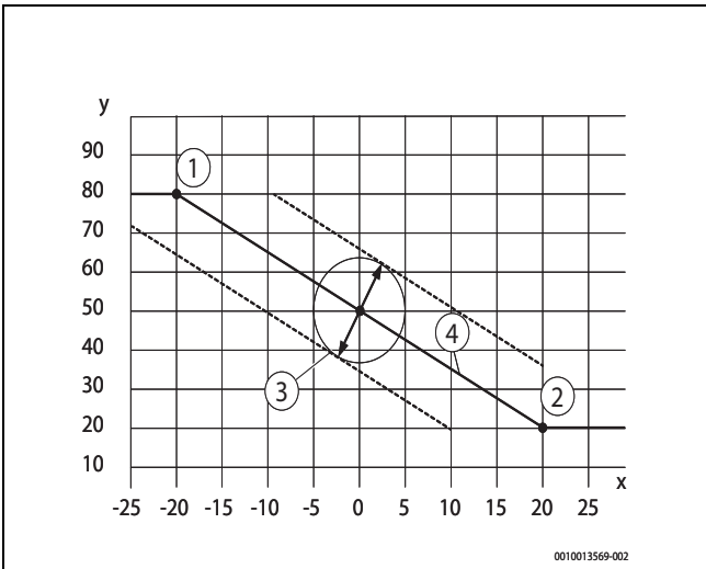
Bild 4 Außentemperaturgeführte Heizkurve
