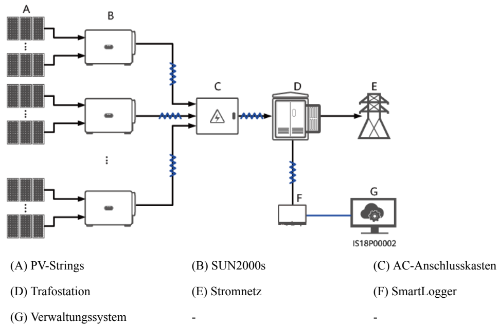
Abbildung 2-2 MBUS-Netzwerkanwendung (ohne SmartMBUS CCO)
