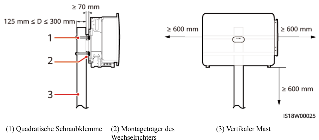
Abbildung 4-16 Montage mit Mastschelle
