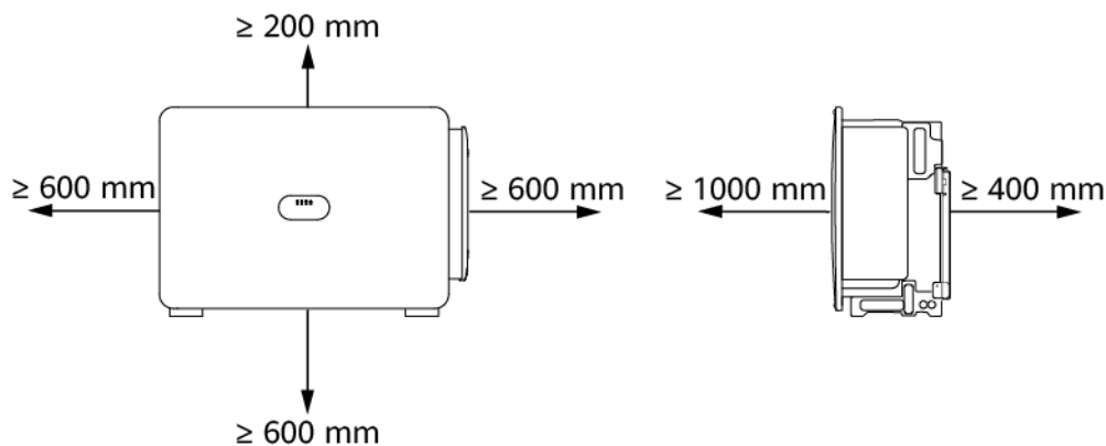
Abbildung 4-4 Abstände
