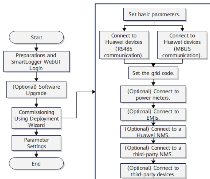
Abbildung 7-2 Inbetriebnahmeprozess mit dem SmartLogger
