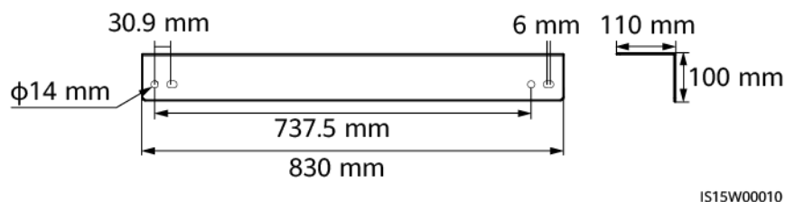
Abbildung 4-8 Empfohlene Luftleitblechabmessungen
