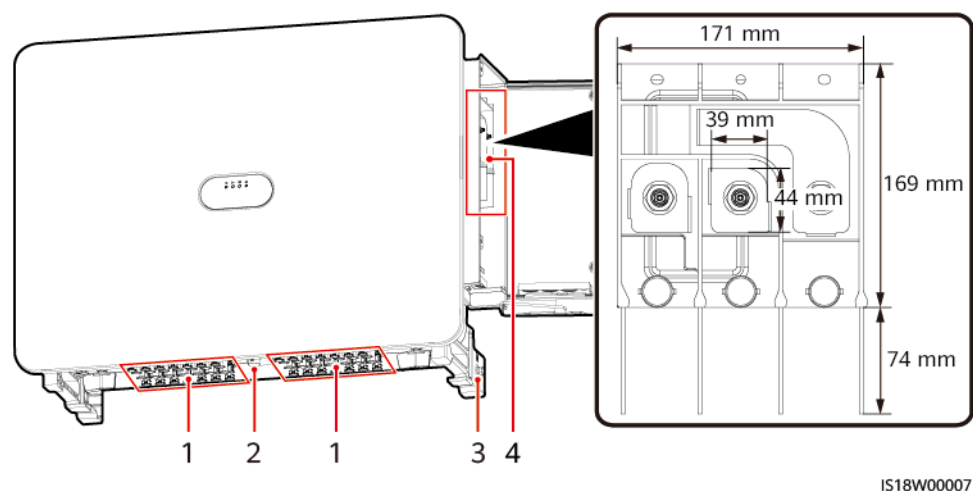
Abbildung 5-4 Verdrahtungsanschlüsse
