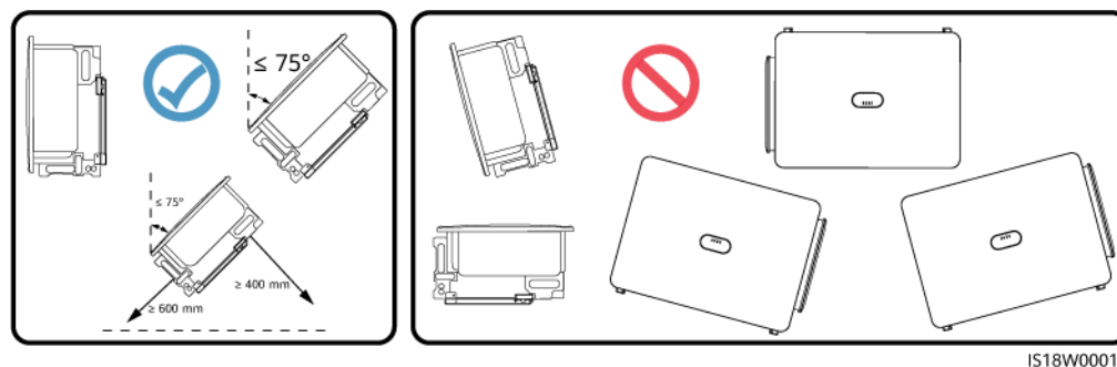
Abbildung 4-10 Montagewinkel
