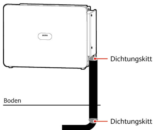
Abbildung 5-14 Installation abgeschlossen
