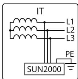
Abbildung 2-6 Stromnetztyp
